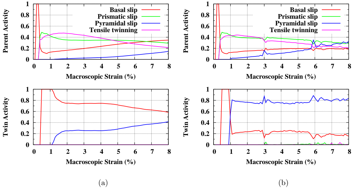
FIGURE 5 – Activités plastiques moyennées des systèmes de déformation principaux de glissement et de maclage au sein des phases maclé et parent obtenues à partir de (a) EPSC et du (b) DI-EPSC.
