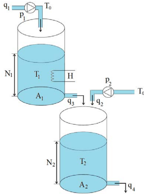
FIGURE 2.1 – Système hydraulique
