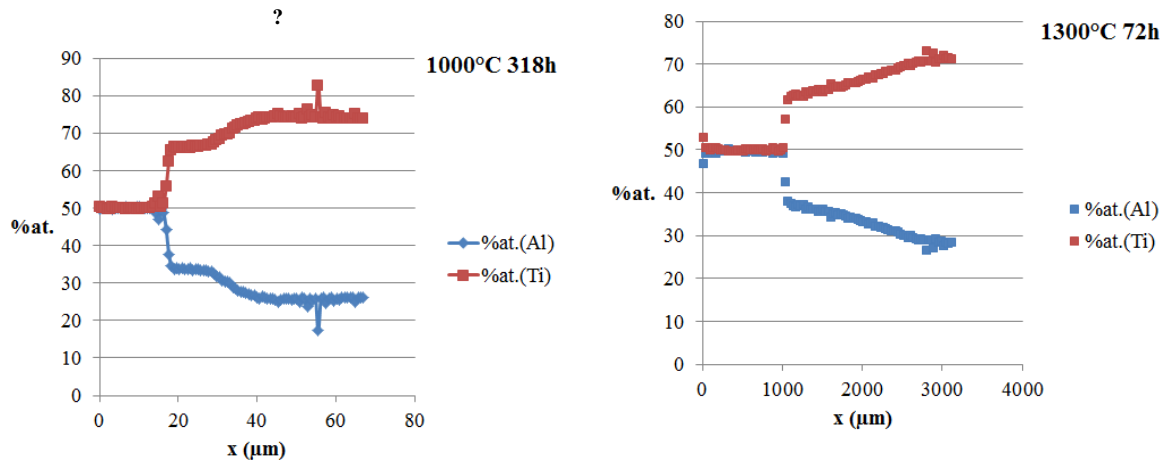
Figure III.12: Profils de concentration en Al mesurés par EDS au MEB après assemblage : à 1000°C pendant 318h (gauche) et 1300°C pendant 72h (droite)
