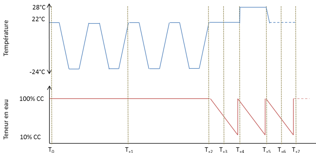
Figure VI-3 : Alternances de modalités climatiques pour la séquence de vieillissement tempéré (Nancy - Cfb), les lignes en tirets représentent des cycles de 24h
