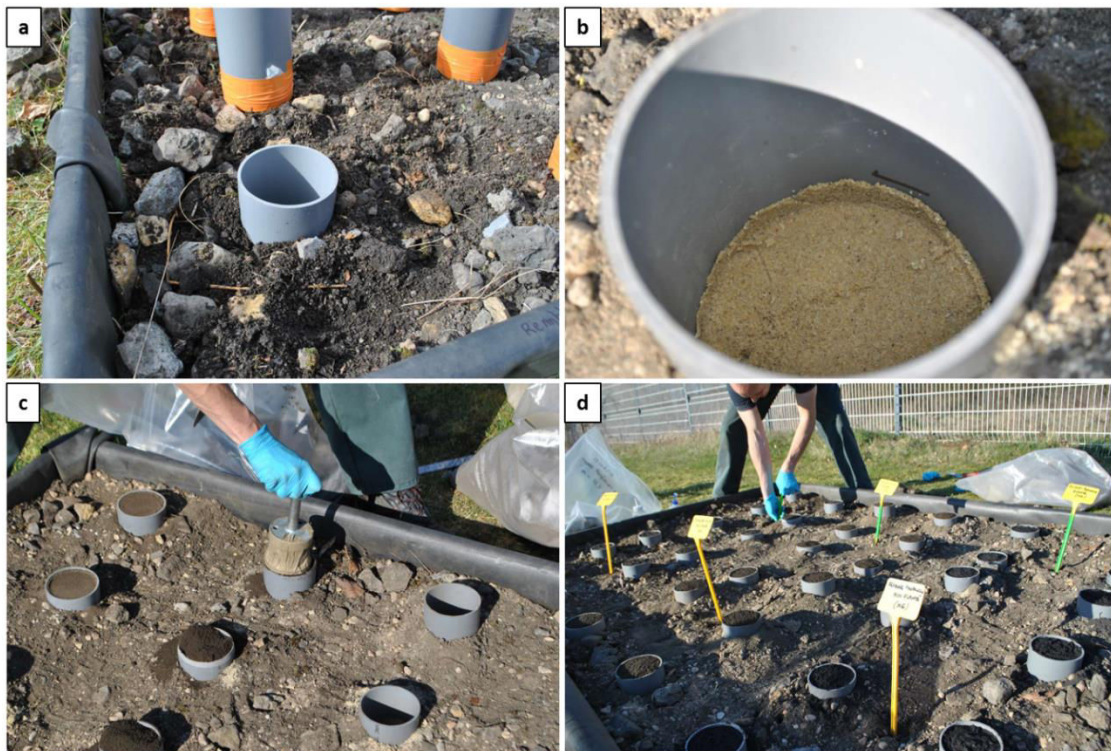
Figure VIII-9 : Photographies de la mise en place des colonnes de suivi de l'atténuation naturelle : (a) implantation des cylindres dans le sol encaissant, (b) dépôt des couches de sable filtrant, (c) tassement à la main du filtre et (d) état global au temps initial
