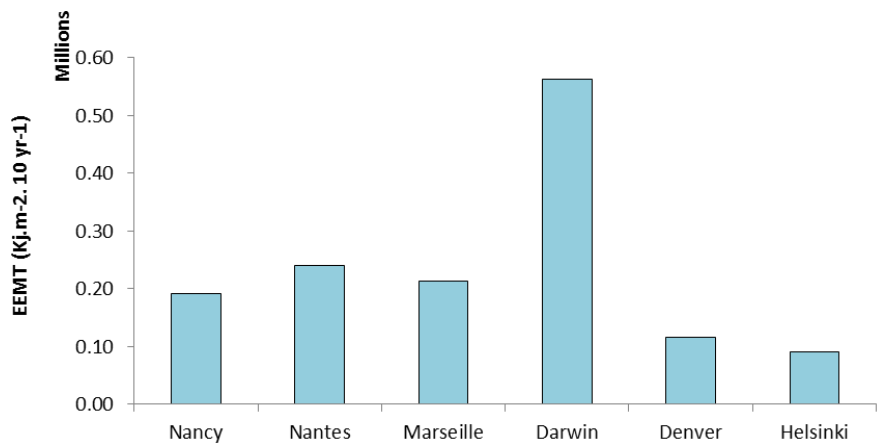
Figure XI-10 : Energies Effectives de Transfert de Masse (EEMT - en \text{Kj m}^{-2} 10\text{ans}^{-1} - Rasmussen et al., 2005; Rasmussen and Tabor, 2007; Runge, 1973) calculées à partir des relevés climatiques actuels des six climats mondiaux
