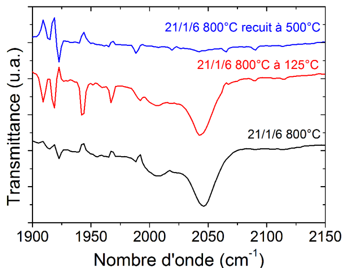
FIGURE 97 – DETAIL DU SPECTRE FTIR DE L'ÉCHANTILLON 21/1/6 BRUT DE DEPOT, A 125°C ET APRES RECUIT
