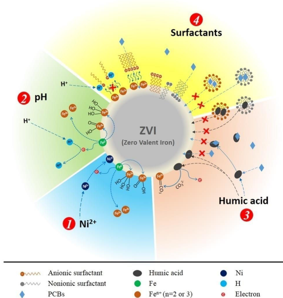
Figure 5. Schéma des influences et effets combinés du tensioactif, de l'acide humique, du pH et de \text{Ni}^{2+} sur la déchloration du PCB-52 par le \text{Fe}^0 .
