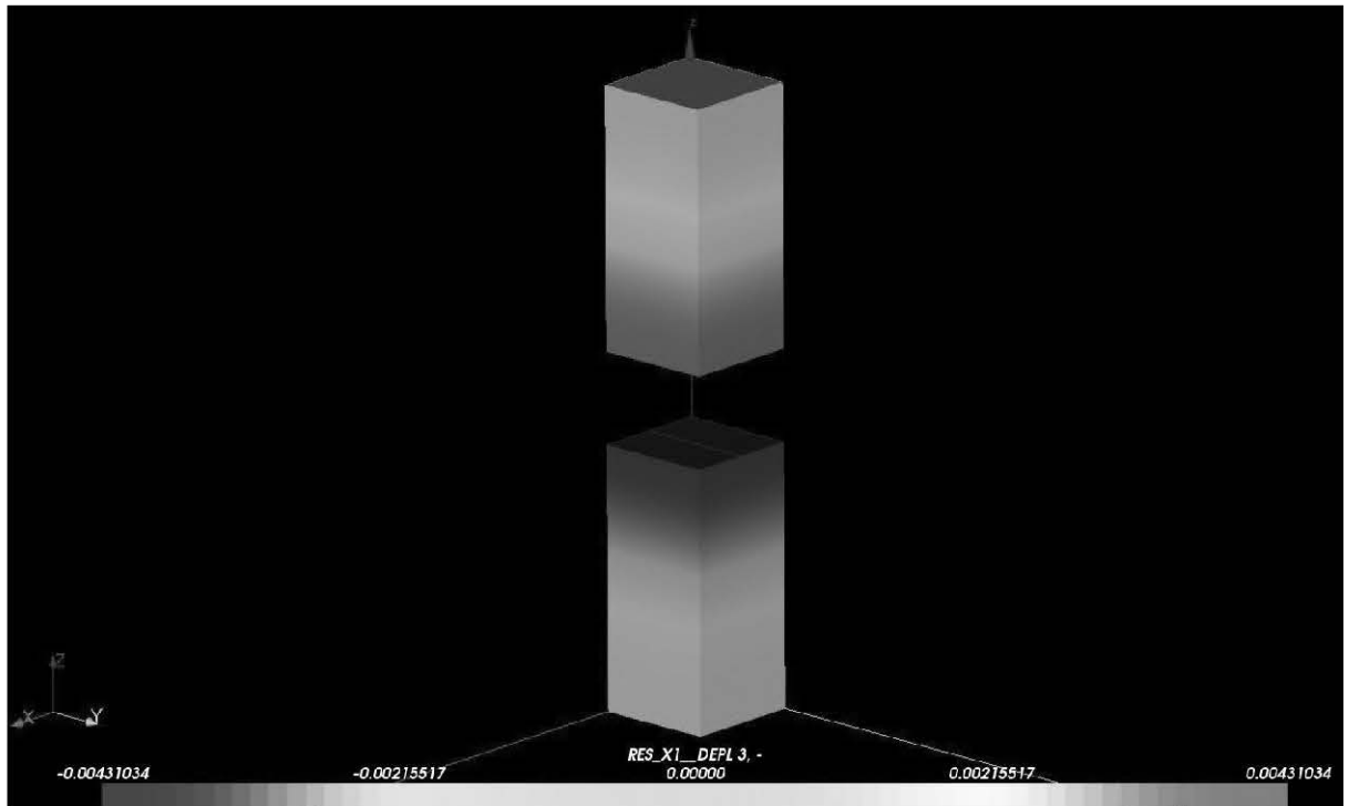
Figure 6.3-a : Champ de déplacements selon la direction (Oz)
