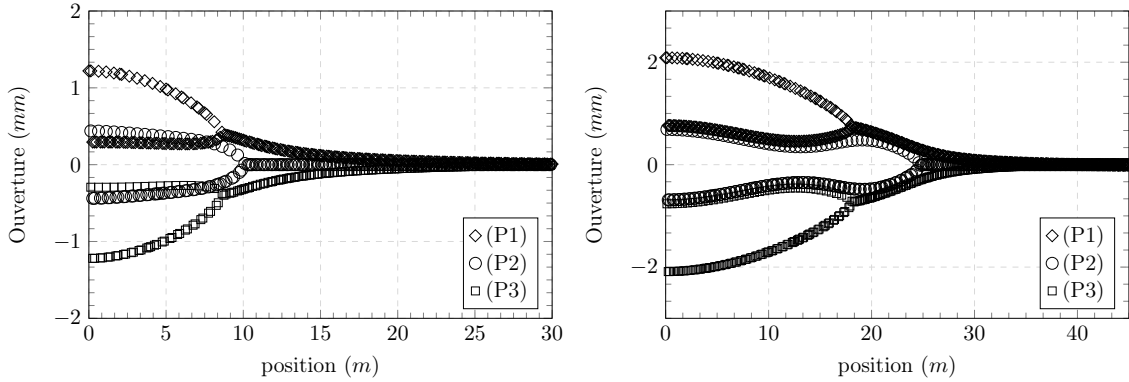
FIGURE 5.15 – Profils des trois fractures pour le cas \mu = 1 \times 10^{-2} \text{ Pa.s} à t_1 = 15\text{s} (gauche) et t_2 = 50\text{s} (droite).
