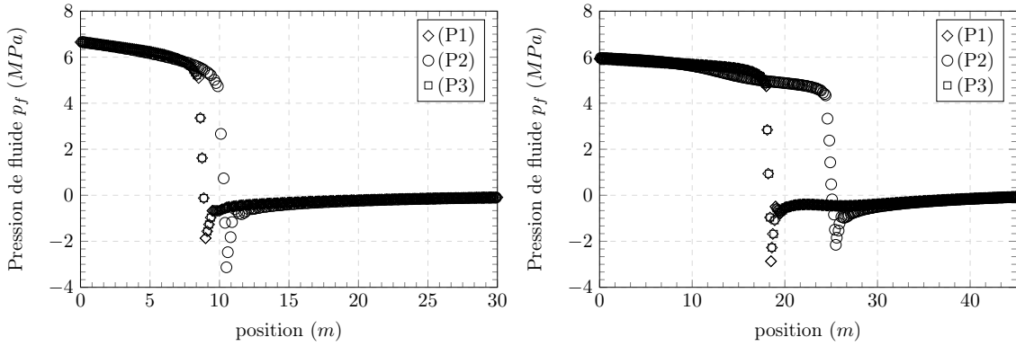
FIGURE 5.16 – Profils de pression de fluide le long des trois fractures pour le cas \mu = 1 \times 10^{-2} \text{ Pa.s} à t_1 = 15\text{s} (gauche) et t_2 = 50\text{s} (droite).
