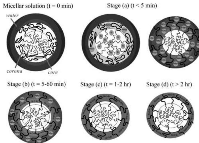
Fig. 2.11 : Modèle proposé pour les premières étapes de formation de SBA-15 ( \text{Si/P123 molaire}=59 ) à l'échelle moléculaire [4].
