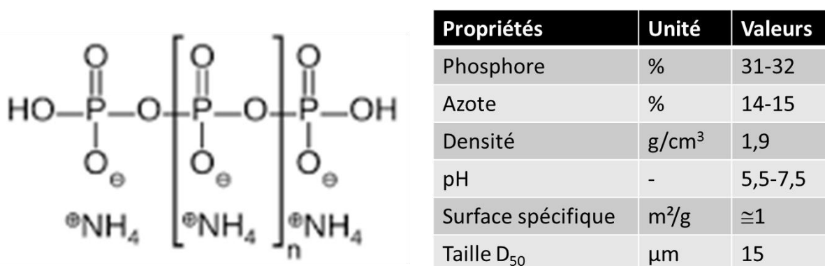
Fig. 2.4 : Structure chimique et caractéristiques de l'AP 422.
