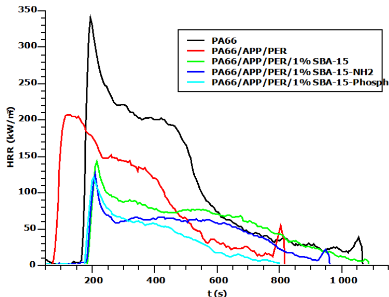
Figure 4.57: Courbes HRR des composites PA66, PA66/APP/PER et PA66/APP/PER/1%( SBA-15, SBA-15-Phosph et SBA-15-NH 2 ) obtenues au cône calorimètre sous une irradiance de 35 kW/m 2 .
