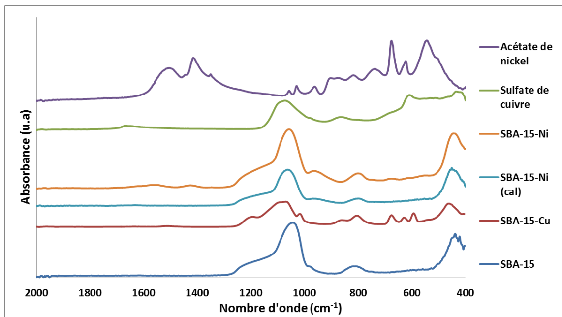
Fig. 3.25 : Spectres ATR des SBA-15 imprégnés par (A) Cu et (B) Ni.
