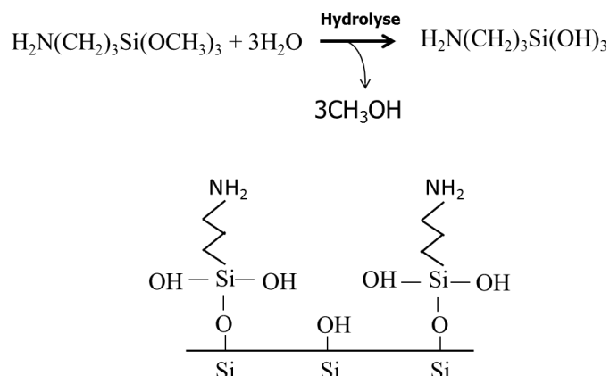
Fig. 3.19 : Interaction entre le SBA-15 et l'APTMS.
