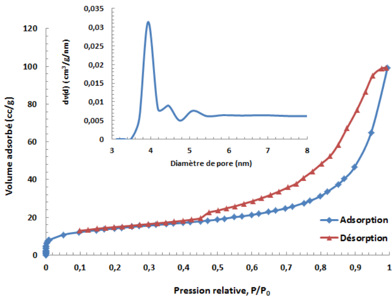
Fig. 3.28 : Isotherme d'adsorption/désorption d'azote d'aluminophosphate calciné et distribution en tailles de pore.
