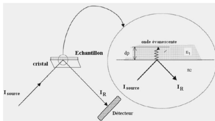
Fig. 2.33 : Schéma du principe de la réflexion totale atténuée (ATR)
