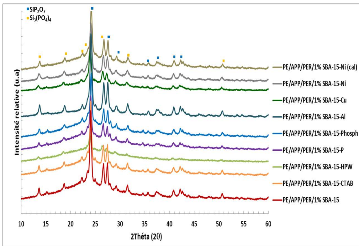
Fig. 4.34 : Diffractogrammes de rayons X après un test au four réalisé sur les composites PE/APP/PER/SBA-15-fonctionnalisés et imprégnés.
