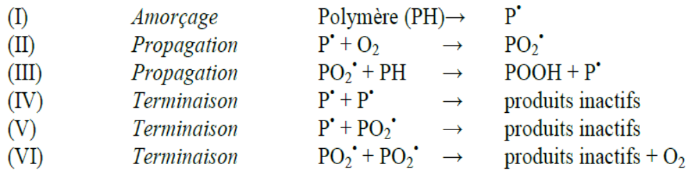
Fig. 1.16 : Le schéma standard d'oxydation des polymères d'après Bolland et Gee [48].
