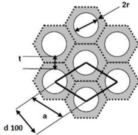
Fig. 2.30 : Schématisation de l'arrangement de pore [37].
