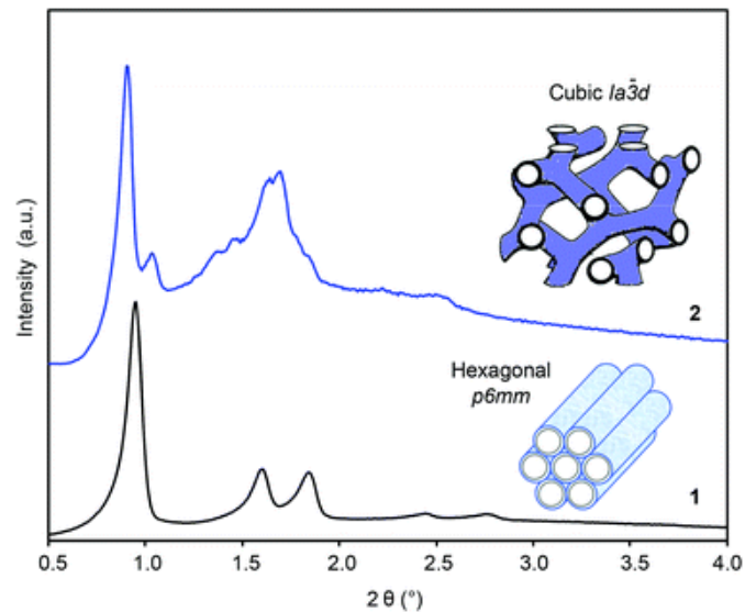
Fig. 2.31 : Diffractogrammes de deux arrangements différents (1) hexagonal et (2) cubique.
