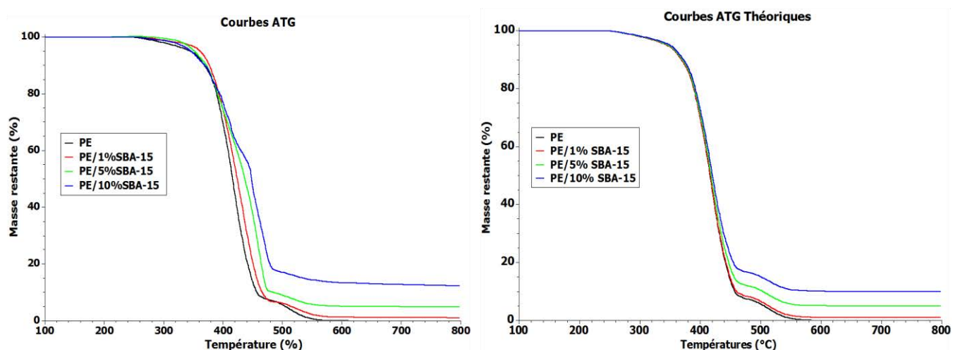
Figure 4.4: Courbes ATG (expérimentales et théoriques) du PE seul et des systèmes PE/ (1, 5 et 10%) SBA-15 avec une vitesse de chauffage de 10^{\circ}C/min sous air.
