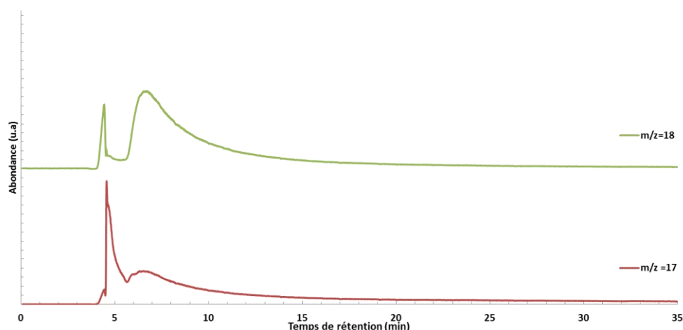
Fig. 3.41 : Chromatogrammes d'eau et d'ammoniac libérés à 600°C par l'APP.
