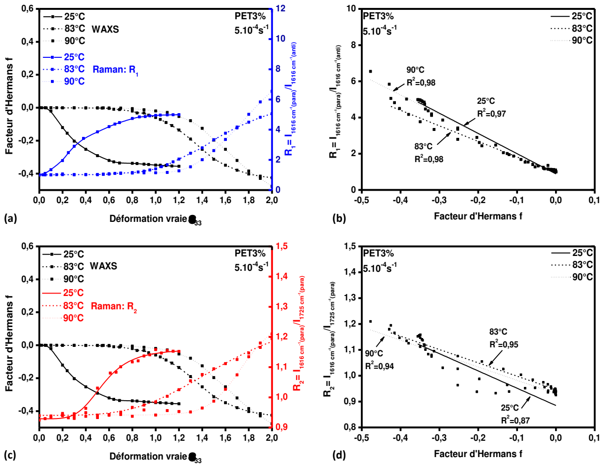
Figure 4.21 : (a) Comparaison entre les évolutions de l'orientation des chaînes macromoléculaires du PET3% déformé en traction uniaxiale à 5.10^{-4}s^{-1} en température ambiante, 83 et 90°C déterminés in situ par WAXS et par spectroscopie Raman. (b) Droites de corrélation entre les deux techniques d'analyse.
