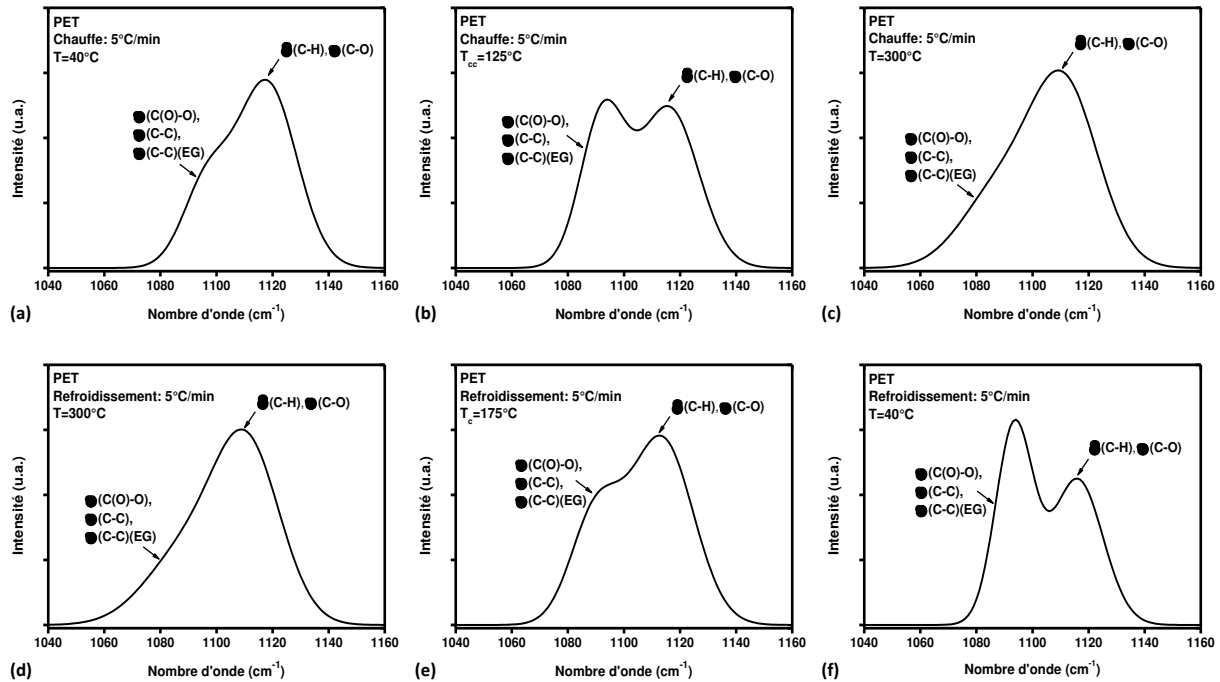
Figure 3.2 : Evolution des bandes vibrationnelles 1096 cm -1 et 1118 cm -1 aux températures (a) 40°C, (b) T_{cc}=125^{\circ}\text{C} et (c) 300°C au cours d'une chauffe et (d) 300°C, (e) T_c=175^{\circ}\text{C} et (f) 40°C au cours d'un refroidissement à 5°C/min.
