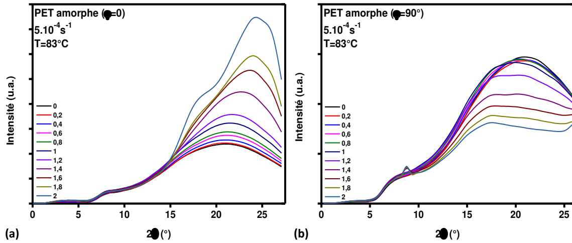
Figure E.4 : Evolution de l'intensité WAXS en fonction de 2\theta pour le PET amorphe déformé à T=83^\circ\text{C} à 5.10^{-4}\text{s}^{-1} . (a) Profil horizontal ( \varphi=0 ) et (b) profil vertical ( \varphi=90^\circ ).
