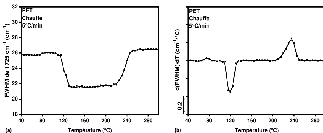
Figure 3.5 : (a) FWHM et (b) sa dérivée par rapport au temps de la bande vibrationnelle à 1725\text{ cm}^{-1} en fonction de la température.
