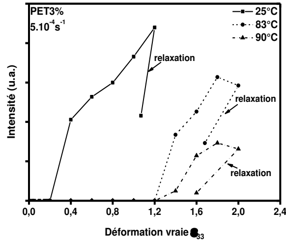
Figure 4.20 : Evolution de l'intensité relative du pic de diffraction de la mésophase (00 \bar{1} ) au cours de la déformation et après relaxation du PET3% sollicité en traction uniaxiale à 5.10^{-4}s^{-1} à 25, 83 et 90°C.
