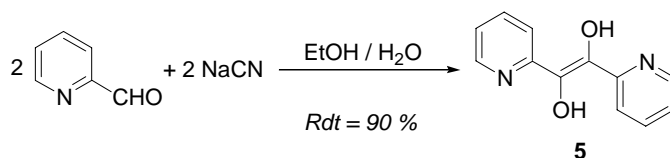
Schéma 12
