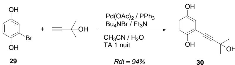
Schéma 72
