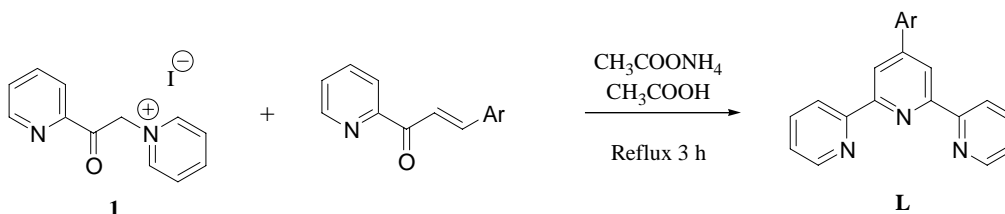
Schéma 7
