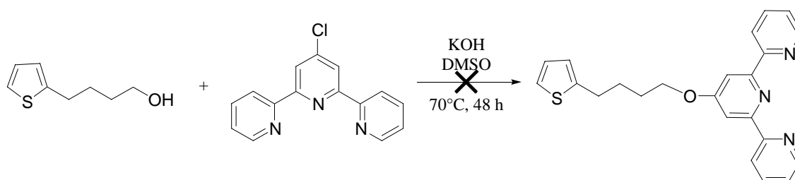
Schéma 43
