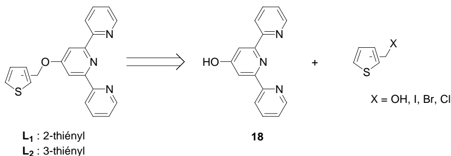
Schéma 46
