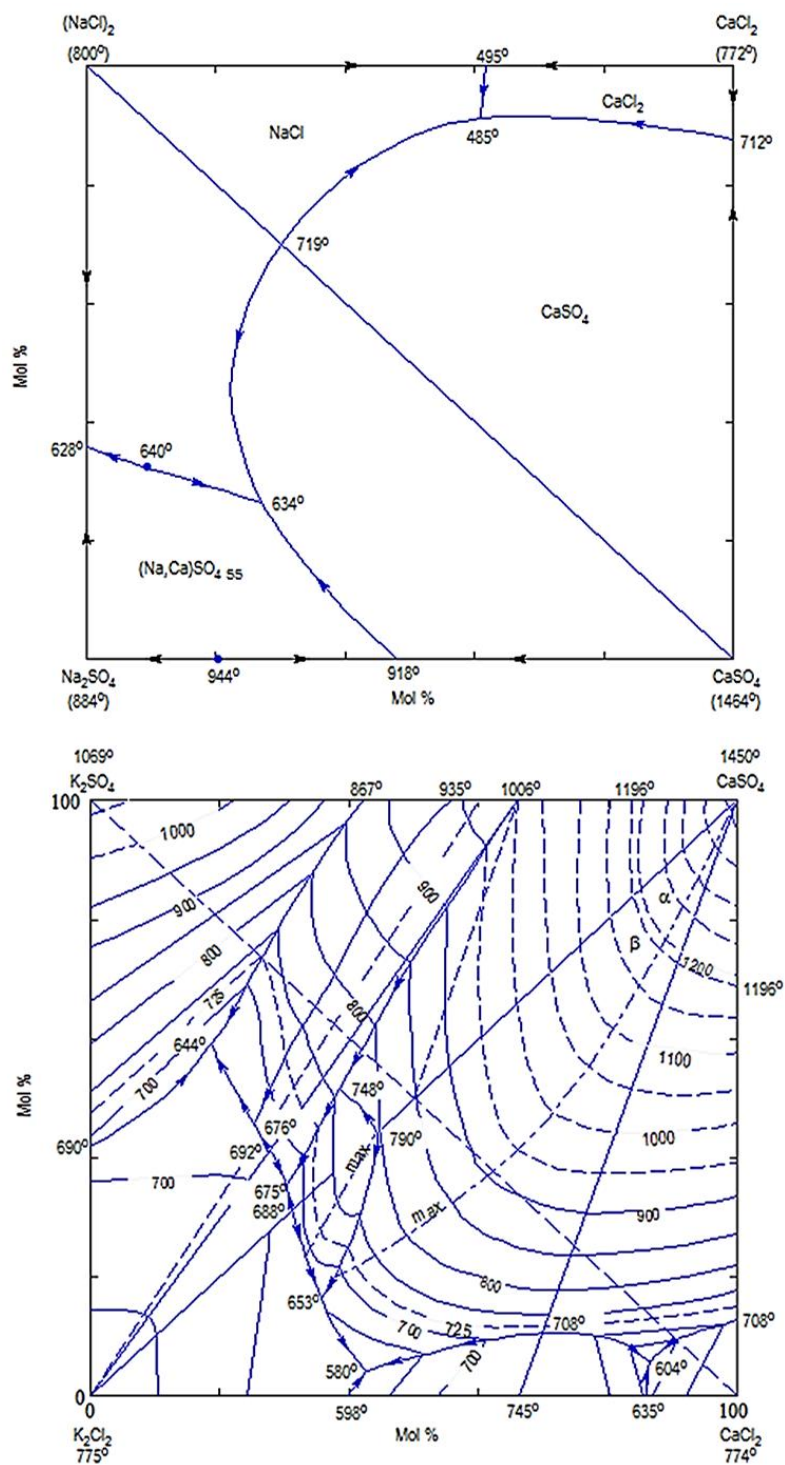
Figure 5 : Nappes liquidus des systèmes (NaCl) 2 - CaCl 2 - Na 2 SO 4 - CaSO 4 [10] et (KCl) 2 - CaCl 2 - K 2 SO 4 - CaSO 4 [23]
