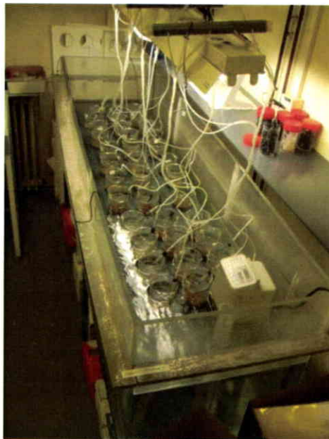
Figure 30. Dispositif expérimental utilisé pour les essais.
