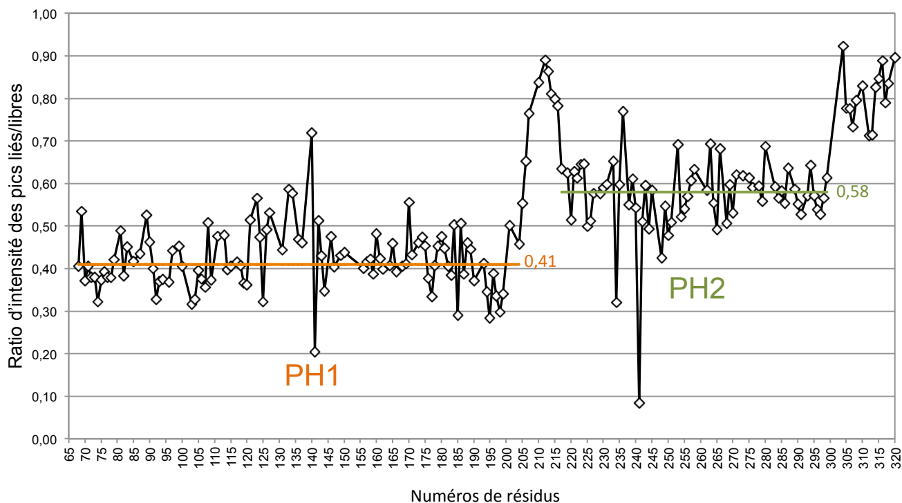
Figure 66. Titration suivie par RMN de la protéine Rtt106(65-320) par la protéine Bcd1(120-303). (A) Comparaison des spectres TROSY-HSQC ^1\text{H} - ^{15}\text{N} obtenus pour la protéine Rtt106(65-320) marquée ^2\text{H} - ^{13}\text{C} - ^{15}\text{N} seule (spectre de gauche) ou en présence de la protéine Bcd1(120-303) ^2\text{H} aux ratios de 0,3 (spectre central) et 1 (spectre de droite). (B) Graphique représentant le ratio d'intensité des pics obtenus pour chaque résidu entre l'expérience TROSY-HSQC ^1\text{H} - ^{15}\text{N} au ratio 0,3 et l'expérience référence. Les droites orange et verte représentent les médianes des valeurs pour les domaines PH1 (résidus 68 à 204) et PH2 (résidus 217 à 299) respectivement. Les deux zones non comprises dans les domaines PH correspondent à la boucle entre les deux domaines (205 à 216) et à l'extension terminale (300 à 320) de la protéine Rtt106.
