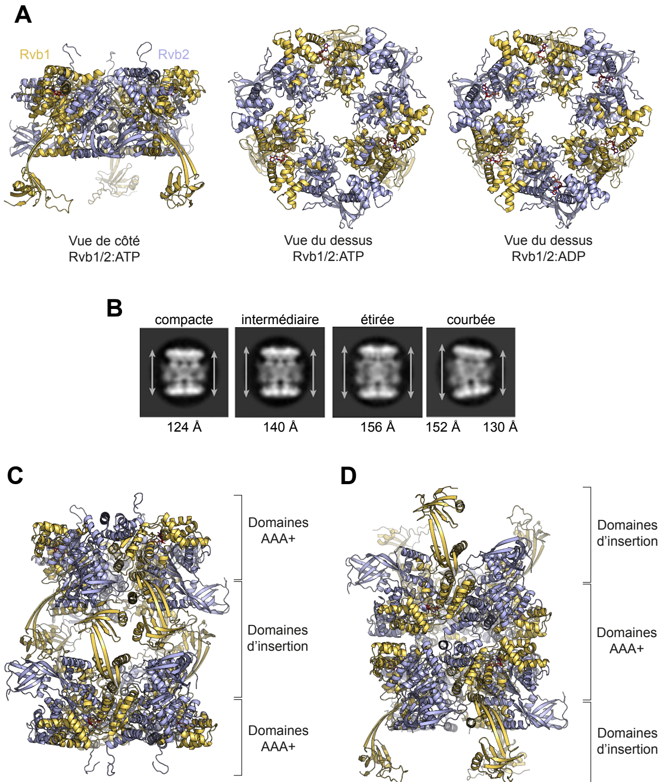
Figure 22. Conformation en hexamère et dodécamère des protéines Rvb1/2. (A) Structure en hexamère des protéines Rvb1/2 de Chaetomium thermophilum (Lakomek et al. , 2015; code PDB : 4WVY). (B) Différentes conformations adoptées par les structures en dodécamères de levure obtenues par cryo-EM (Ewens et al. , 2016). (C) Structure en dodécamère des protéines Rvb1/2 (Lakomek et al. , 2015; code PDB : 4WVY) avec interaction entre les hexamères par les domaines d'insertion ou (D) par les domaines AAA+ (anneau).
