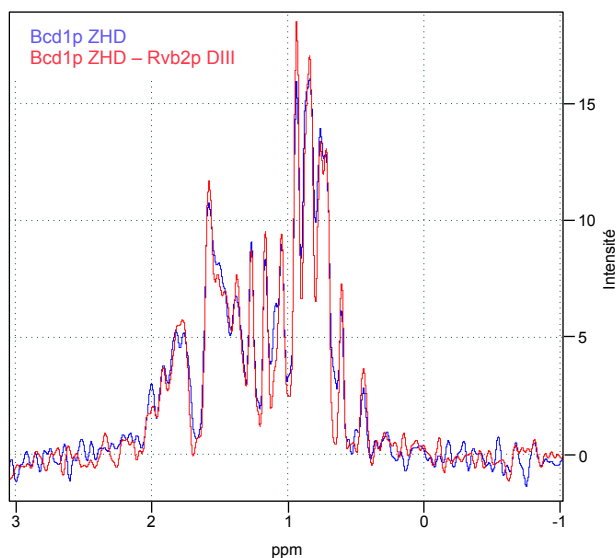
Figure 47. Tests d'interaction suivis par RMN entre le ZHD de Bcd1p et les domaines DII et DIII de Rvb2p. Les spectres RMN 1D présentés ont été enregistrés sur les protons portés par des atomes ^{13}\text{C} dont le déplacement chimique se situe entre 2 ppm et -1 ppm (groupements méthyle) avec le logiciel TopSpin 3.0. Comme pour la figure 41, la courbe bleue représente la protéine marquée au ^{13}\text{C} et la courbe rouge cette même protéine supplémentée d'une autre non-marquée entre lesquelles est testée l'interaction. (A) ZHD de Bcd1p sans (bleu) et avec (rouge) Rvb2p DII ext . (B) ZHD de Bcd1p sans (bleu) et avec (rouge) Rvb2p DIII.
