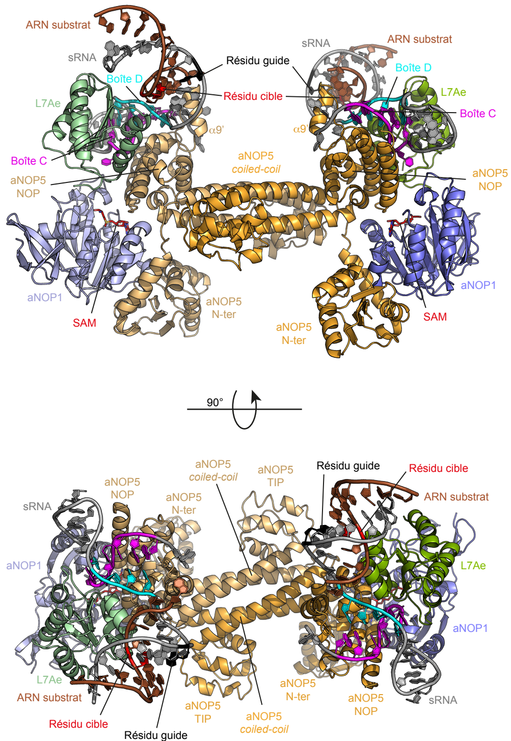
Figure 13. Structure tridimensionnelle d'une sRNP de l'archée Pyrococcus furiosus avec deux demi-sRNA C/D et avec le substrat en vue de côté (haut) ou du dessus (bas). Cette structure a été obtenue par cristallographie aux rayons X (Xue et al. , 2010 ; code PDB : 3NMU). Les résidus colorés en noir sur la structure du sRNA (ARN guide) correspondent aux 5 èmes résidus en amont des boîtes D, devant servir de guide à la 2'-O-méthylation de l'ARN substrat. Les résidus de l'ARN cible colorés en rouge correspondent aux résidus cibles devant accepter le transfert d'un groupement méthyle.
