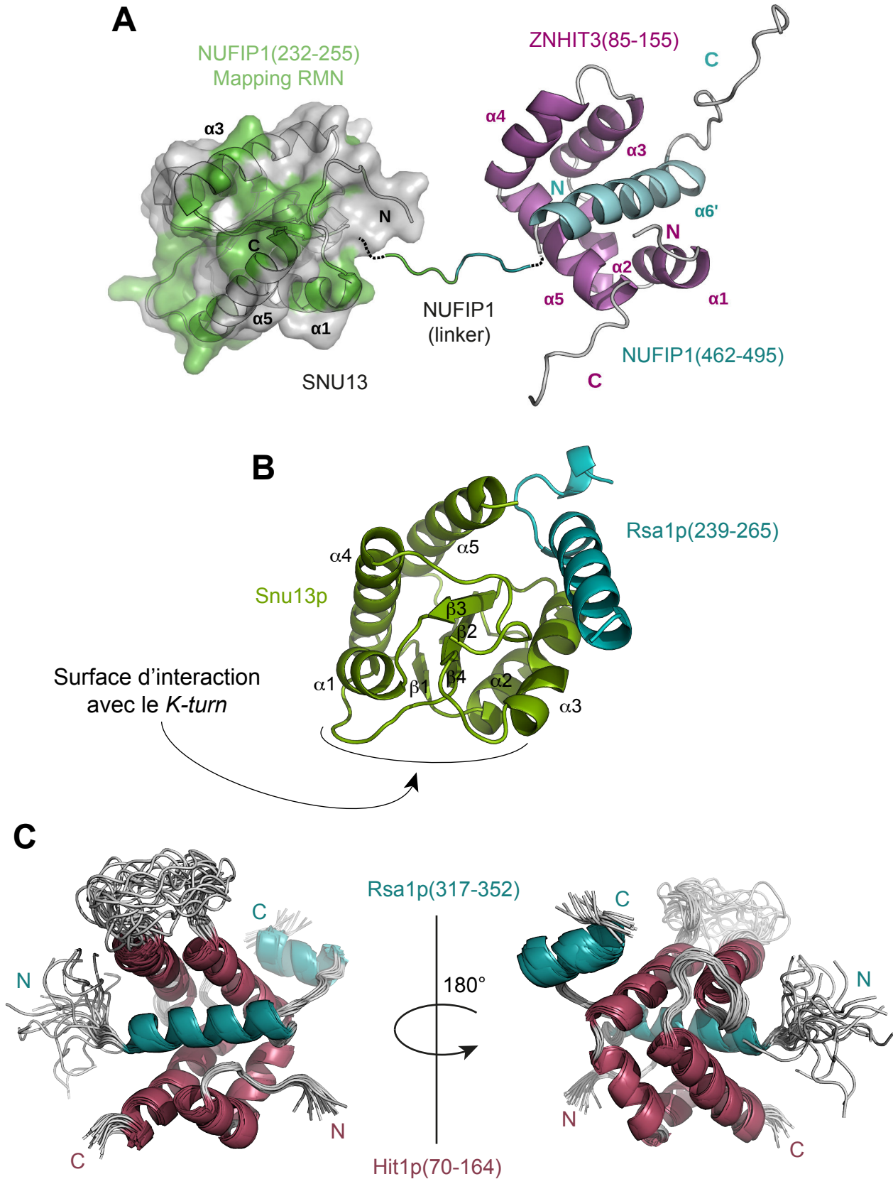
Figure 25. Structures tridimensionnelles des complexes entre les protéines Rsa1/NUFIP1 et Snu13/SNU13 ou Rsa1/NUFIP1 et Hit1/ZNHIT3. (A) Structure 3D du complexe NUFIP1(462-495):ZNHIT3(85-155) (à droite) et cartographie par RMN des résidus touchés par l'interaction de NUFIP1 sur SNU13 (d'après Quinternet et al. , 2016; code PDB : 5L85). (B) Structure 3D du complexe Rsa1p(239-265):Snu13p (Bizarro et al. , 2014; code PDB : 4NUT). (C) Structure 3D du complexe Rsa1p(317-352):Hit1p(70-164) (d'après Rothé, Saliou et al. , 2014; code PDB : 2MJF).
