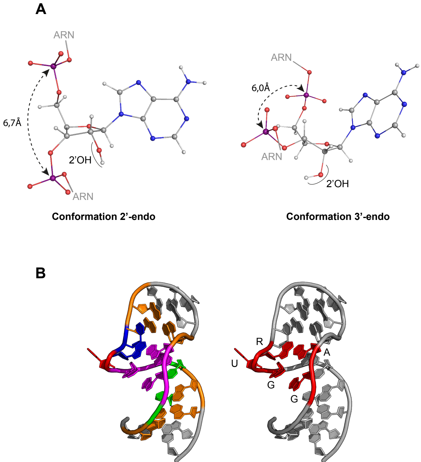
Figure 6. 5 nucléotides de l'ARN en K-turn ou K-loop ont une conformation de type 2'-endo. (A) Représentation des conformations 2'-endo (à gauche) et 3'-endo (à droite) du ribose d'un résidu adénosine. Les deux distances indiquées séparent les deux groupements phosphate encadrant le nucléoside (les atomes de phosphate sont colorés en violet). (B) Report sur la structure de l'ARN (le code couleur de la représentation de gauche correspond à celui de la figure 3) des 5 résidus annotés possédant une conformation 2'-endo (en rouge sur la représentation de droite).
