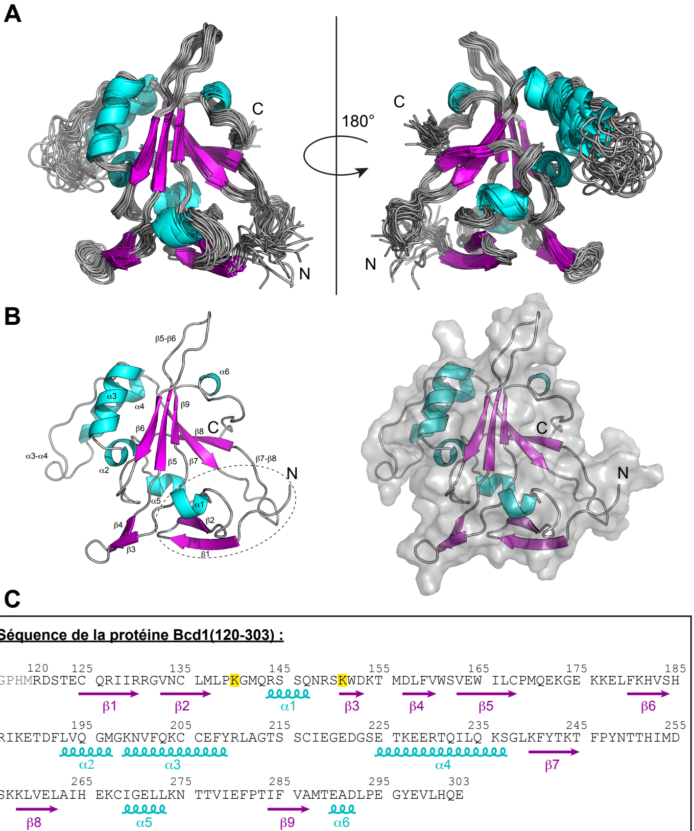
Figure 70. Structure 3D en solution de la protéine Bcd1(120-303). (A) Superposition des 20 structures calculées avec CYANA présentant la plus basse énergie, représentées en cartoon, avec coloration des structures secondaires. Les hélices \alpha sont colorées en cyan et les brins \beta en magenta. (B) Représentation uniquement de la structure de plus basse énergie, avec annotation des différents éléments de structure secondaire (à gauche) et dans l'enveloppe de surface (à droite). Les régions annotées \beta 5-\beta 6 , \alpha 3-\alpha 4 et \beta 7-\beta 8 correspondent à des boucles. La région encadrée en pointillés correspond à la séquence 120-149. (C) Séquence de la protéine Bcd1(120-303) avec report des éléments de structure secondaire en dessous. Les quatre premiers résidus (GPHM, en gris et non numérotés) correspondent aux résidus de l'étiquette 6xHistidines restants après coupure par la 3C. La séquence de la protéine débute au résidu R120. Les résidus surlignés en jaune correspondent aux lysines réalisant des ponts avec Rtt106p lors des expériences de cross-link.
