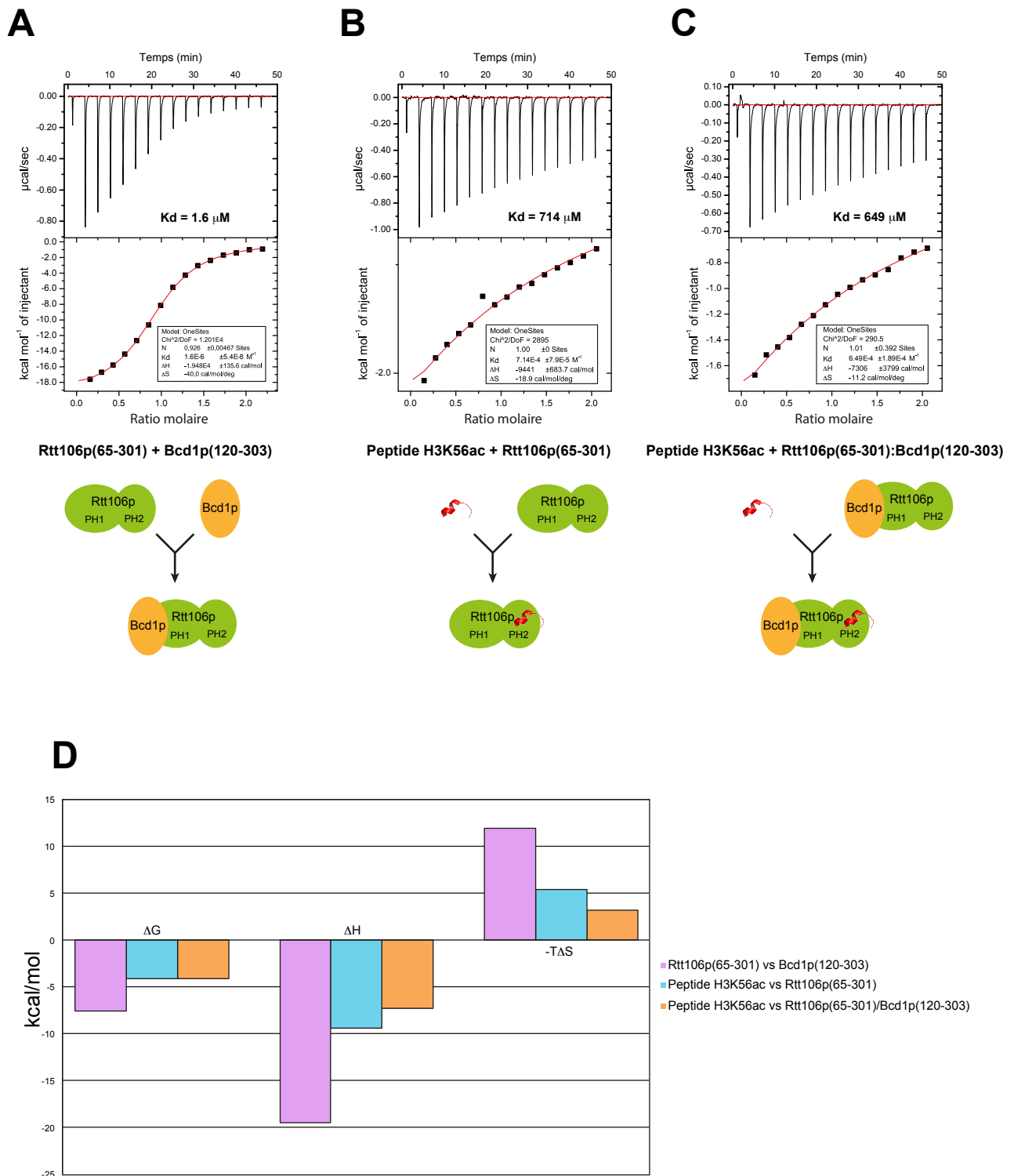
Figure 78. Possibilité d'un complexe à trois partenaires entre Bcd1p, Rtt106p et un peptide de l'histone H3. Résultats d'ITC entre (A) les protéines Rtt106(65-301) et Bcd1(120-303), (B) le peptide H3K56ac et la protéine Rtt106(65-301) et (C) le peptide H3K56ac et le complexe Rtt106p(65-301):Bcd1p(120-303). Dans les expériences (B) et (C) le peptide est placé dans la seringue à une concentration de 2 mM et le partenaire testé est placé dans la cuve à une concentration de 200 µM. Les schémas sous les résultats d'ITC représentent les complexes formés lors des différentes expériences. (D) Paramètres thermodynamiques enregistrés lors des trois expériences ITC (A), (B) et (C).
