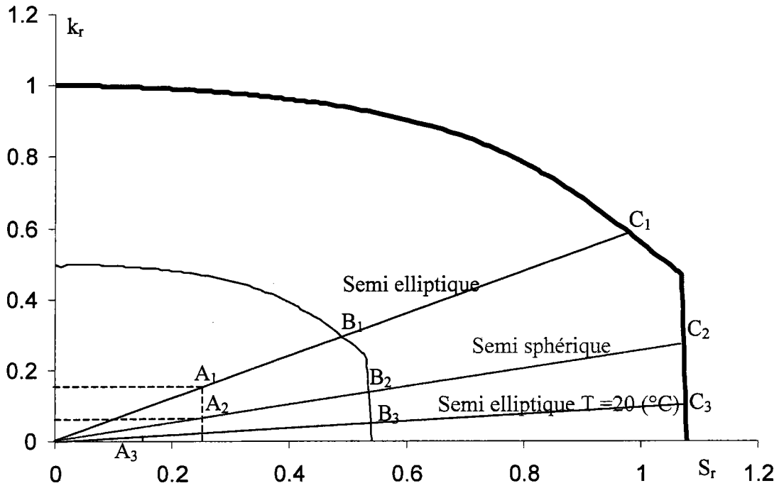
Figure N° VI-11 Facteur de sécurité et de fiabilité obtenu par la méthode déterministe pour les trois cas étudiés à la température de 20°C
