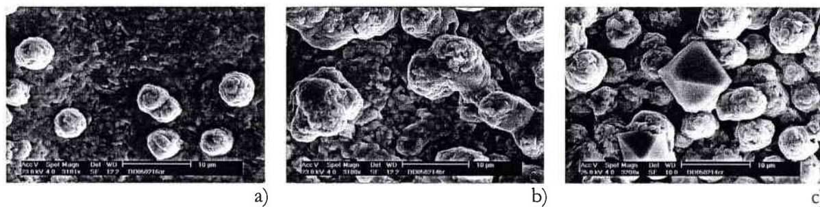
Figure 86 : Représentation de la morphologie des films électrodéposés en fonction de l'épaisseur - ([Bi]+[Sb])/[Te] = 1 - [Sb]/[Bi] = 8 - [Te] = 10^2 M - a) e = 2 \mu m - b) e = 4 \mu m - c) e = 6 \mu m .
