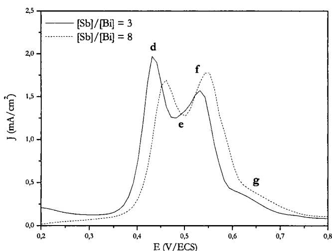
Figure 65 : Comportement électrochimique, après un balayage cathodique, d'une solution ternaire de rapport ([Bi] + [Sb])/[Te] = 1 , en milieu perchlorique 1 M, tartrique 0,1 M - [Te] = 10^{-2} M - E_{base} = 0,1 V/ECS, Incrément = 10 mV, Electrode de travail : Au - T_{on} = T_{off} = 5 s.
