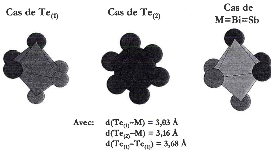
Figure 6 : Environnement atomique des atomes du composé (\text{Bi}_{1-x}\text{Sb}_x)_2\text{Te}_3 .
