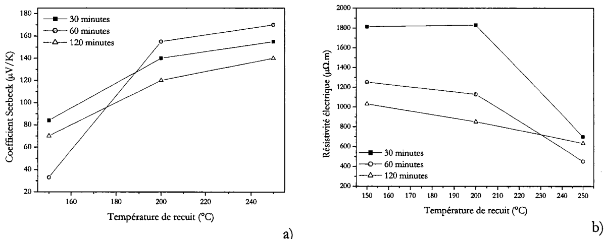
Figure 54 : Evolution des propriétés thermoélectriques de composés électrodéposés (\text{Bi}_{1-x}\text{Sb}_x)_2\text{Te}_3 en fonction de la température et de la durée d'un recuit réalisé sous argon – ([\text{Bi}]+[\text{Sb}])/[\text{Te}] = 1 , [\text{Sb}]/[\text{Bi}] = 3 , E = -0,17 \text{ V}/\text{ECS} , [\text{Te}] = 10^2 \text{ M} – a) Coefficient Seebeck \alpha , b) Résistivité électrique \rho .
