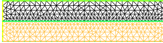
FIG. 3.1 – Maillage de domaine avec \Gamma_c = ]0, 4[ \times \{\frac{1}{2}\} .
