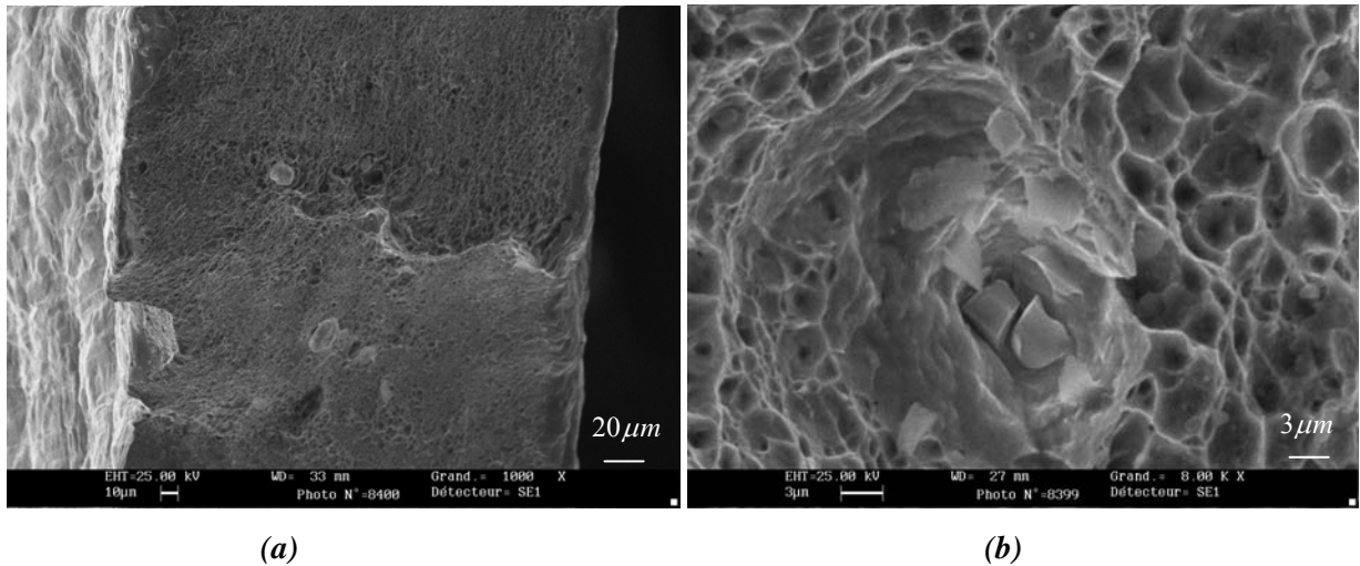
Figure II.37. Faciès de rupture en traction uniaxiale d'un échantillon d'acier 304. Observation de la rupture en (a), décohésion et rupture fragile d'une inclusion de forme rectangulaire en (b)
