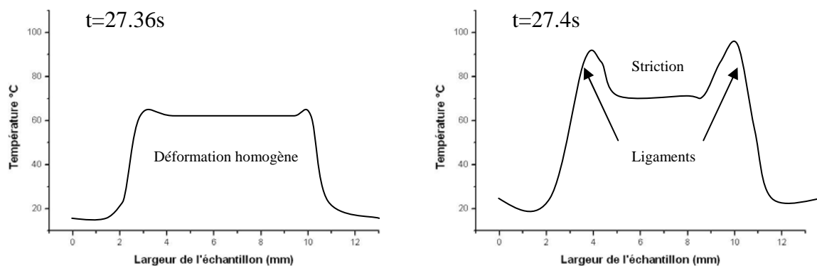
Figure I.21. Evolution du profil de température au sein de la striction durant un essai de traction quasi-statique d'un acier TRIP 800
