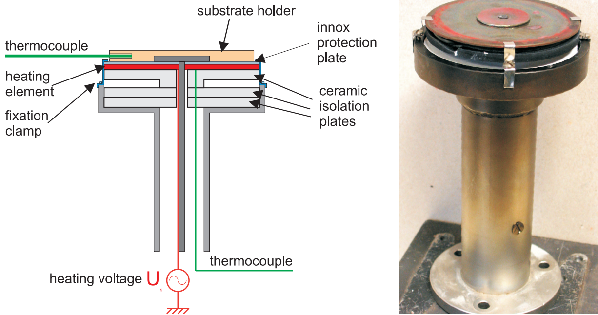
Fig. 2.9: La tour porte-substrat. La photographie montre la tour sans la partie porte-substrat.
