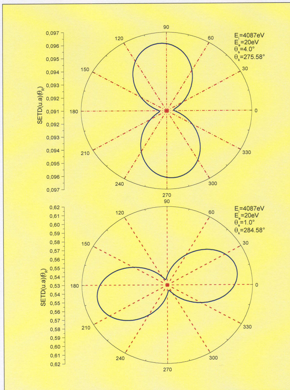
Figure 8 : variation de la SETD de l'ionisation de H_2 en fonction de l'angle polaire \theta_R (intégration sur toutes les directions de l'électron éjecté) pour E_i = 4087\text{eV} , E_e = 20\text{eV} et pour \theta_s = 1.0^\circ , 4.0^\circ .
