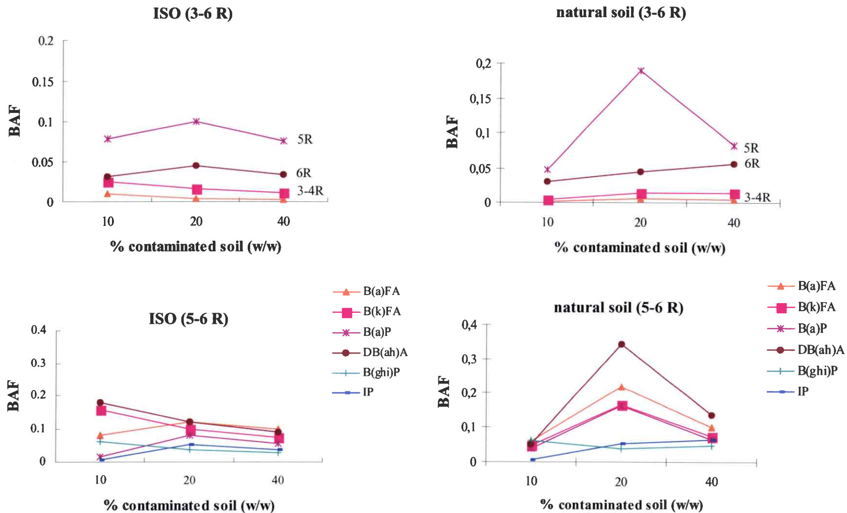
Fig. V. Comparaison des facteurs de bioaccumulation (BAF) des HAP dans les vers de terre juvéniles exposés 24 semaines à différentes concentrations (10%, 20%, 40%) du sol contaminé mélangé au sol contrôle ISO ou au sol naturel.
