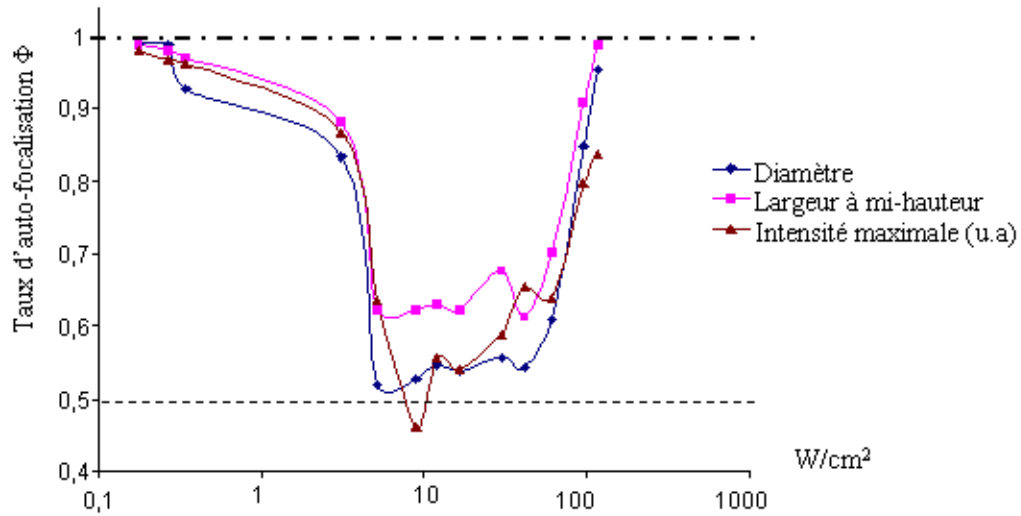
FIG. 5.2 – Évolution du taux d’auto-focalisation en fonction de l’intensité à l’état stationnaire pour un waist w = 25 \mu m à \lambda = 1.56 \mu m à la température T = 20^0C . La ligne horizontale correspond à une égalité entre le diamètre d’entrée et de sortie du faisceau, caractéristique du soliton spatial : les profils d’entrée et de sortie sont identiques.
