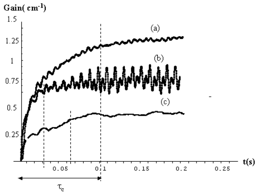
FIG. 3.27 – Gain dynamique à 15^{\circ}\text{C} pour différentes intensités : (a) 62 \text{ mW}/\text{cm}^2 , (b) 97 \text{ mW}/\text{cm}^2 , (c) 28 \text{ mW}/\text{cm}^2 .
