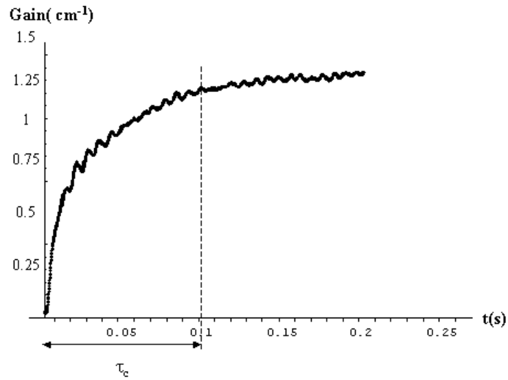
FIG. 3.26 – Gain dynamique à 15^{\circ}\text{C} pour une intensité de 62 \text{ mW}/\text{cm}^2 .
