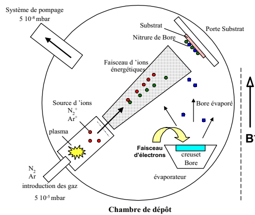
Figure 4: Représentation schématique d'un bâti de dépôt par IBAD
