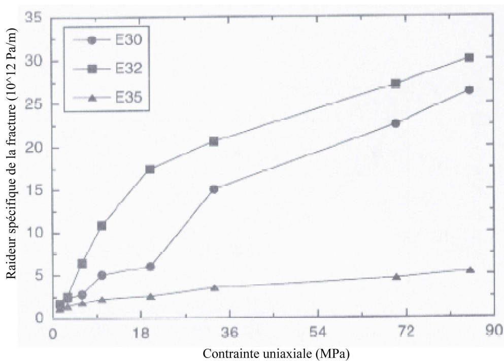
Figure 123 : Variation de la raideur spécifique en fonction de la contrainte normale à la fracture pour trois échantillons de granite de Stripa (Pyrak-Nolte (1996)).
