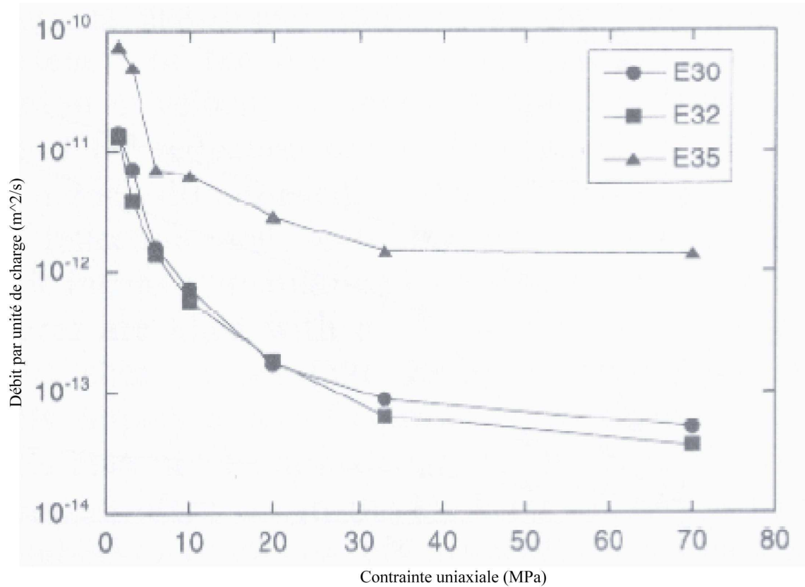
Figure 122 : Le débit de fluide par unité de charge en fonction de la contrainte appliquée perpendiculairement à une seule fracture pour trois échantillons de granite (Stripa granite) (Pyrak-Nolte, 1996).
