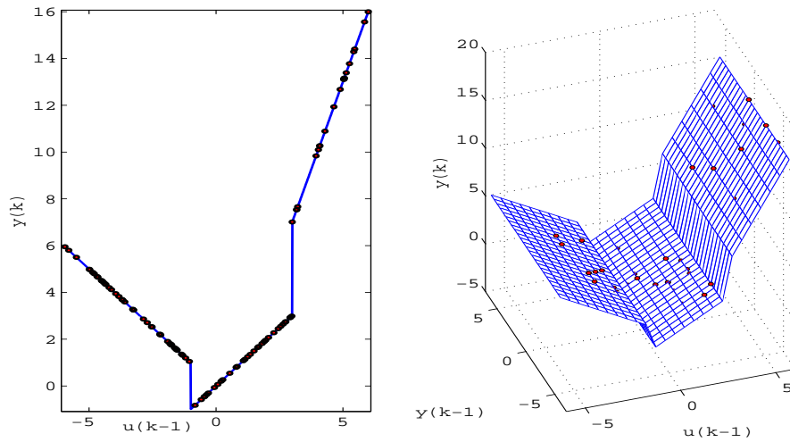
FIG. 1.9: Exemple de modèle PWARX
