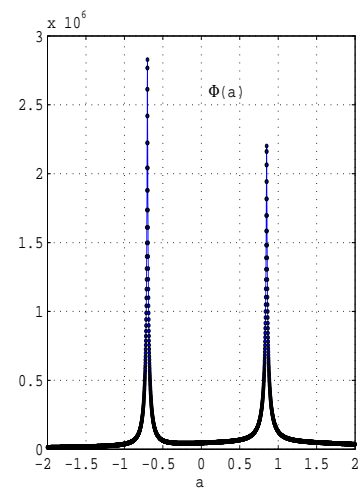
FIG. 1.17: Fonction coût
