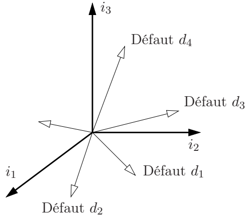
FIG. 2.2: Résidus directionnels
