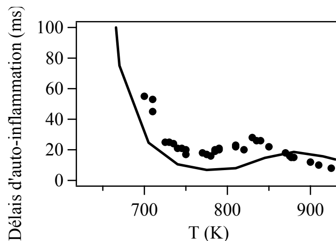
Figure IV-6 : Délais d'auto-inflammation de mélanges stœchiométriques 2-méthylpentane/oxygène/azote/argon en machine à compression rapide (Griffiths et al. , 1997b) de 6 à 10 bar, pour une pression initiale de 300 Torr et une charge de 131 \text{ mol/m}^3 .
