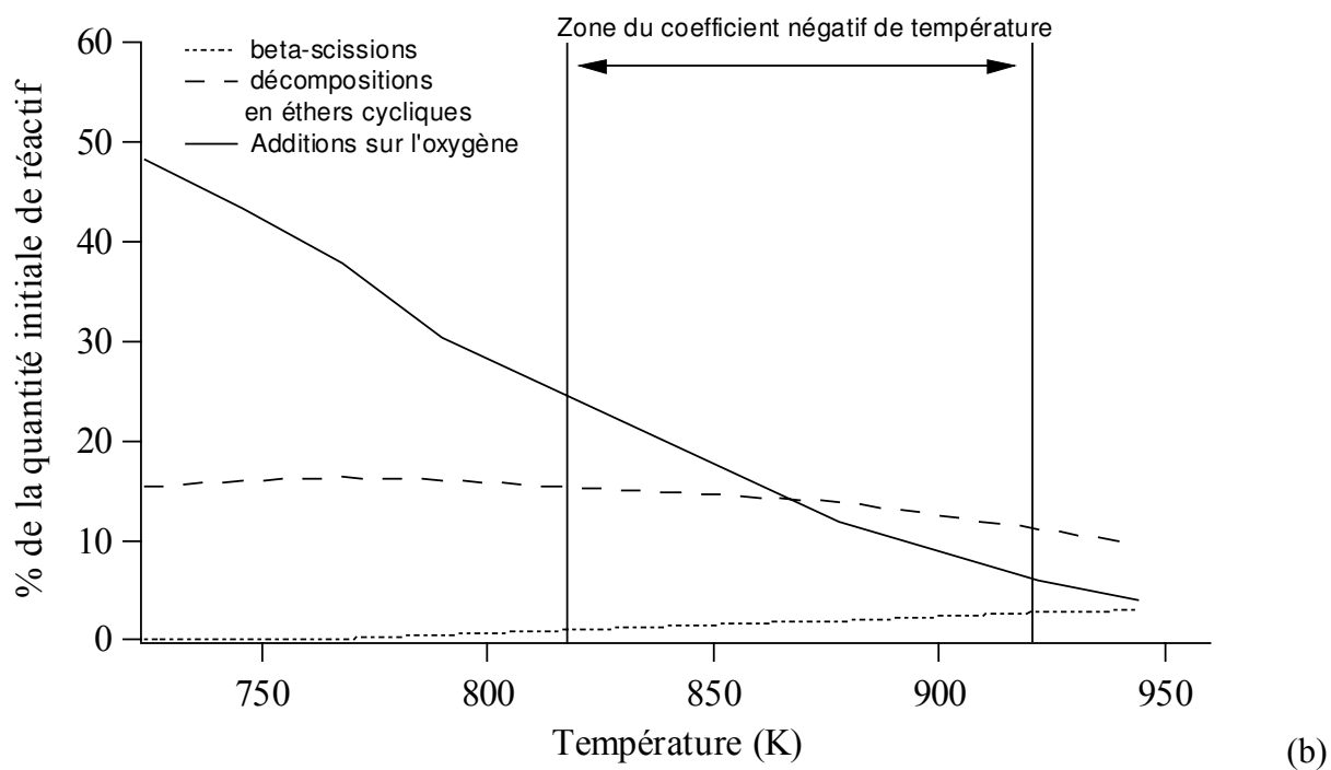
Figure IV-19 : Evolution en fonction de la température des flux en pourcentage de la consommation de réactif pour le n -heptane par type de réactions (a) des radicaux R\bullet et (b) des radicaux \bullet QOOH .
