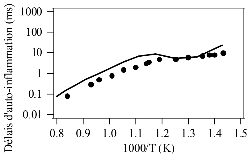
Figure IV-12 : Délais d'auto-inflammation de mélanges stœchiométriques iso-octane/air en fonction de la température en tube à onde de choc (Fieweger et al. , 1997) à 40 bar et une richesse de 1.
