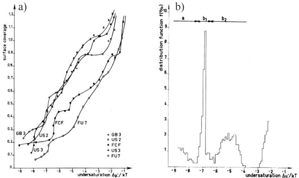
Figure 1.3. : a) Isotherme d'adsorption de tensioactif alkyldodecylammonium sur différents échantillons des kaolinites à 25°C. b) Courbe de distribution des énergies d'adsorption d'alkyldodecylammonium sur la kaolinite GB3 (Cunin 1977 ; Cases et al., 1986).
