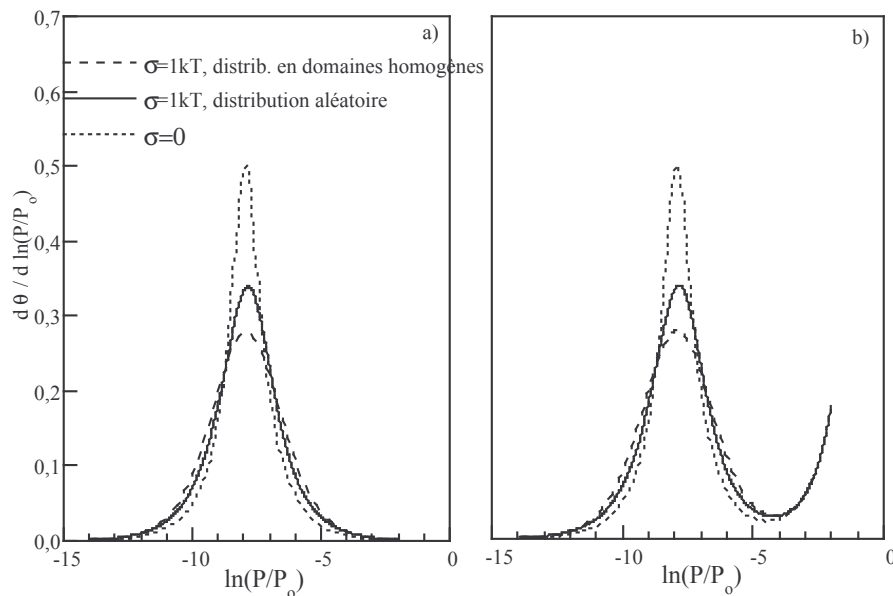
Figure A.3. : Isothermes dérivées calculées à partir de l'équation (I.2.) pour une fonction de distribution \chi gaussienne ( C_0 = 1000 ) des énergies d'adsorption en considérant l'arrangement des sites aléatoire ou en domaines homogènes. La courbe \sigma=0 correspond à l'isotherme locale initiale ( \omega_0=2kT ) - a) adsorption limitée à une couche et b) adsorption multicouche.
