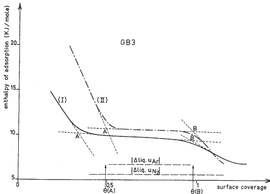
Figure I.4. : Enthalpie d'adsorption d'argon (I) et N_2 (II) à 77K en fonction du taux de recouvrement de la surface de la kaolinite GB3 (Cases et al. , 1986).
