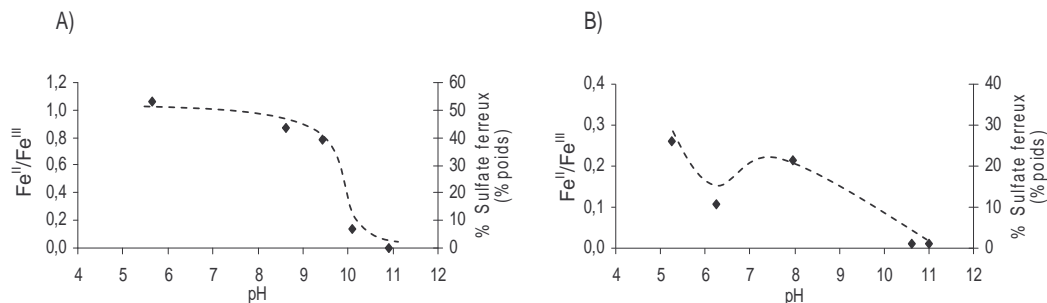
Figure 3.6 : Variation du rapport \text{Fe}^{\text{II}}/\text{Fe}^{\text{III}} des sulfates superficiels d'une pyrite conditionnée à différents pH avec du NaOH en solution (A : fraction granulométrique 32-63 \mu\text{m} , B : fraction granulométrique 0-150 \mu\text{m} )
