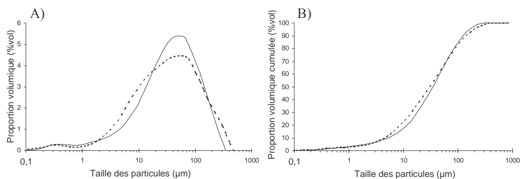
Figure 6.1 : Distribution granulométrique du matériel étudié (courbe pleine) et du rejet de concentrateur de référence (courbe hachurée) : histogramme (A) et courbe cumulée (B)
