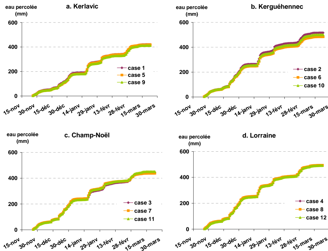
Figures 3.2.1 : Hauteurs d'eau percolée cumulées des 4 sols du dispositif (période de suivi 2002-03)
