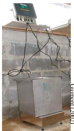
Photo 2.4.1 : Bac de récupération des percolats équipé d'une balance reliée à une interface d'enregistrement
