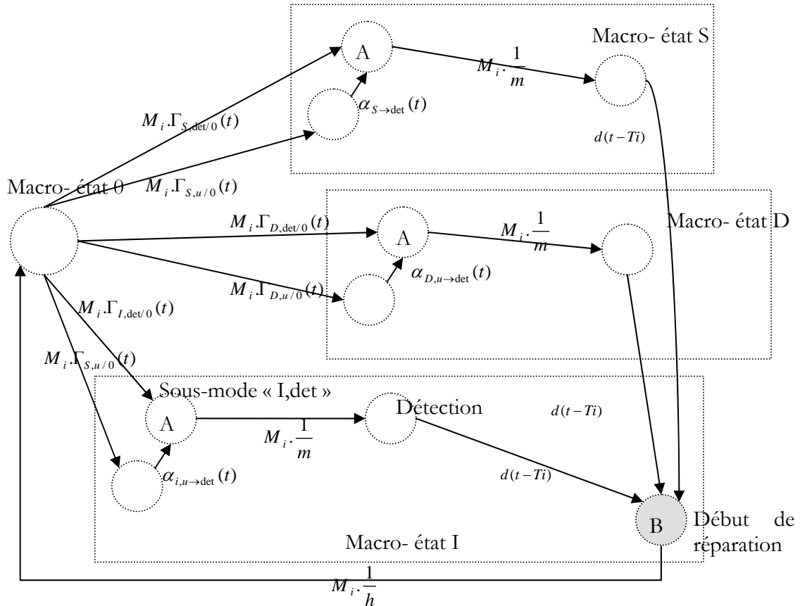
Figure 38: Chaîne de Markov équivalente en dehors des périodes de maintenance
