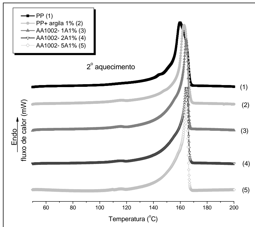
Figura 5.4.4: Termogramas de DSC para amostras de PP e PP (nano)compósitos com 1% em massa de argila organofílica preparados com o compatibilizante AA1002: a) resfriamento b) 2º aquecimento.
