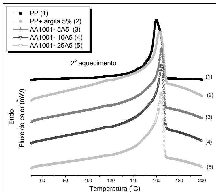
Figura 5.4.6: Termogramas de 2 o aquecimento para amostras de PP e PP (nano)compósitos com 5% em massa de argila organofílica preparados com o compatibilizante AA1001.
