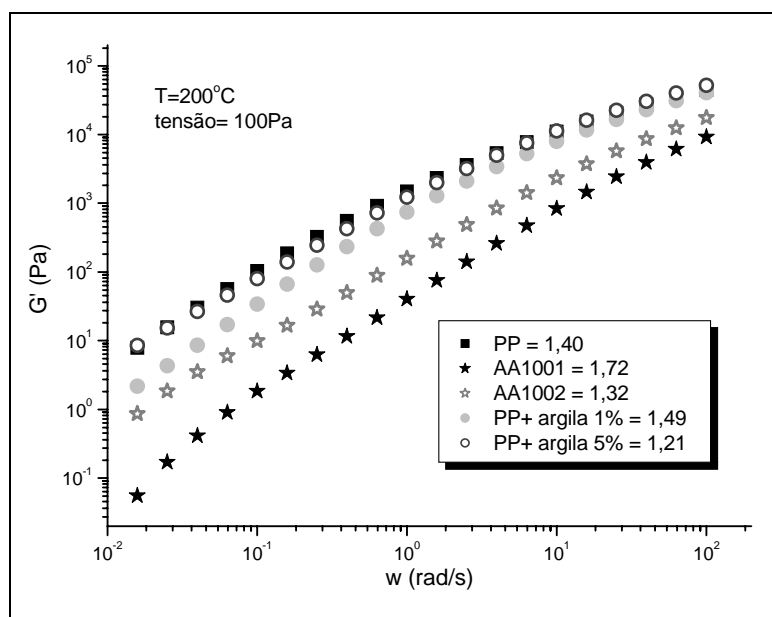
Figura 5.7.2: Gráfico de G' por freqüência para o PP, os compatibilizantes AA1001 e AA1002 puros e as amostras preparadas com 1 e 5 % em massa de argila organofílica. Detalhe da inclinação de cada uma das curvas na região de 0,02 a 0,1 rad/s.
