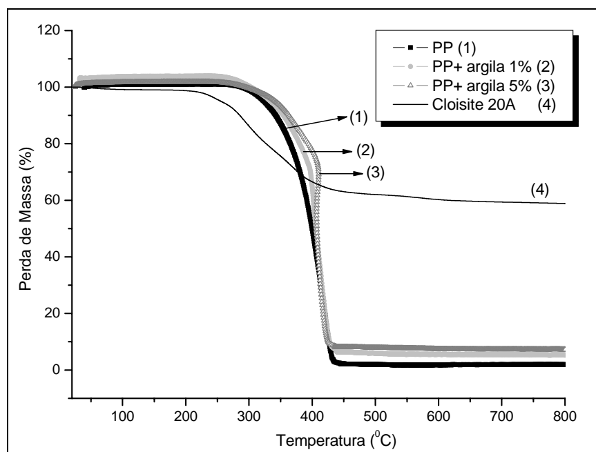
Figura 5.3.1: Curvas de TGA comparativas para a argila organofílica, o polipropileno e misturas de polipropileno com 1 e 5 % em massa de argila.
