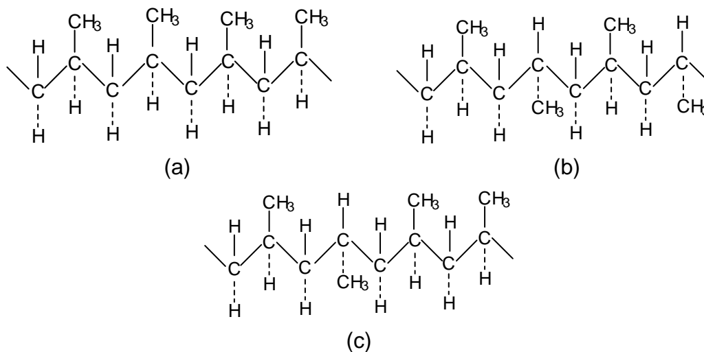
Figura 2.1.3: Configurações do polipropileno segundo sua taticidade: a) isotático, b) sindiotático, c) atático.
