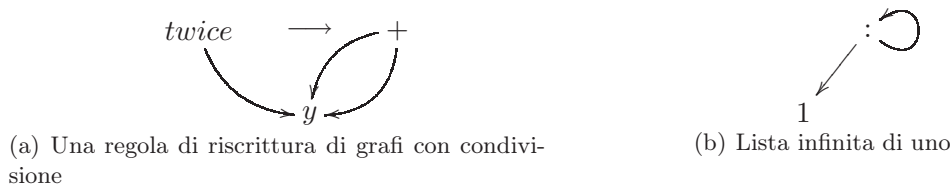
Figure 1: Esempi di termini-grafi
