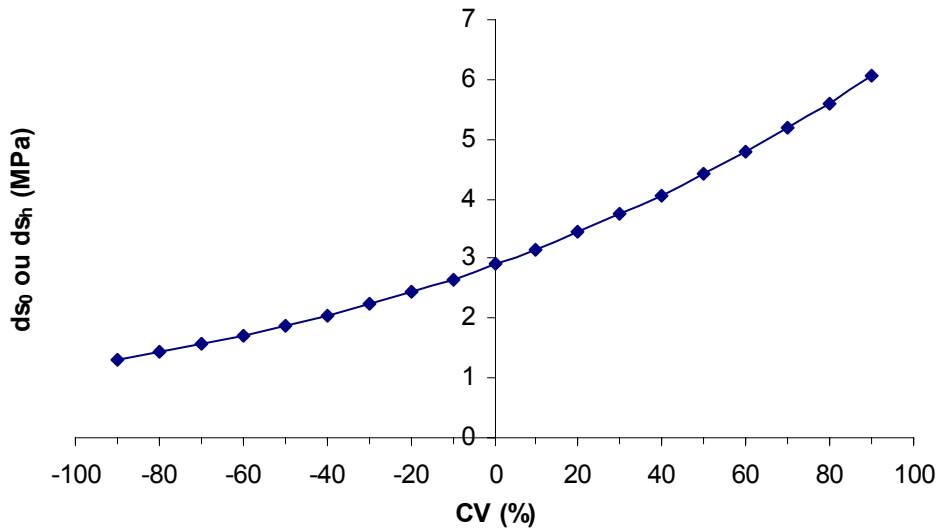
Figure IV.21 - Influence du paramètre n_D sur l'incrément de déplacement de deux paramètres d'écroûissage
