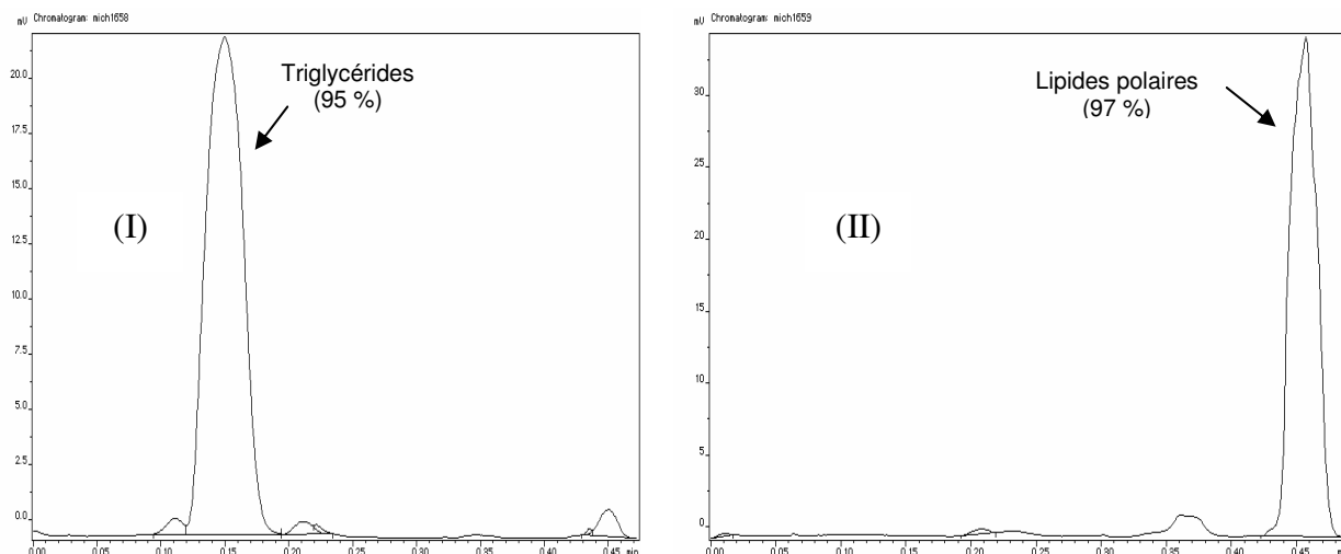
Figure IV.24. Analyse par CCM Iatroscan ® des fractions de (I) lipides neutres et de (II) lipides polaires séparées sur une colonne d'acide silicique, éluant : hexane / éther diéthylique / acide formique (80 / 20 / 0,2 ; v / v / v).
