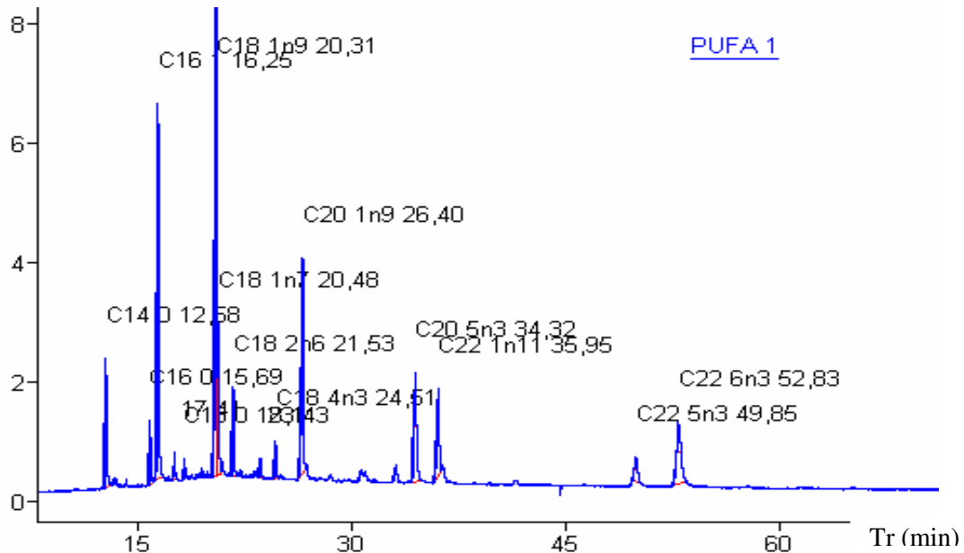
Figure 1. Chromatogramme des acides gras du PUFA 1, analysé par chromatographie en phase gazeuse Péri 2000 (Périchrom) sur une colonne capillaire (25 m de longueur, 0,25 mm de diamètre, 0,5 \mu\text{m} d'épaisseur du film) de polyéthylène glycol dopé avec de l'acide téréphtalique.
