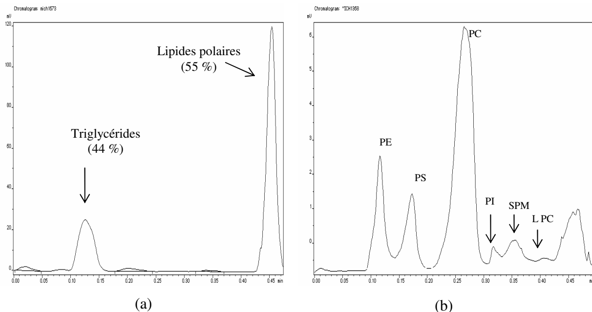
Figure IV.21. Séparation par CCM Iatroscan ® des classes de lipides et des phospholipides de l’huile des culots protéiques issus de l’hydrolyse enzymatique ; (a) séparation dans l’éluant : hexane / éther diéthylique / acide formique (80 / 20 / 0,2, v / v / v) ; (b) séparation du pic de lipides polaires dans l’éluant : chloroforme / méthanol / eau / ammoniacque 25 % (47 / 20 / 2,5 / 0,28, v / v / v / v) ; l’échantillon a été dissous à raison de 5 mg / ml de mélange chloroforme / méthanol (2 / 1, v / v). PE : phosphatidyléthanoline, PC : phosphatidylcholine, SPM : sphingomyéline LPC : lyso-phosphatidylcholine, PS : phosphatidylsérine, PI : phosphatidylinositol.
