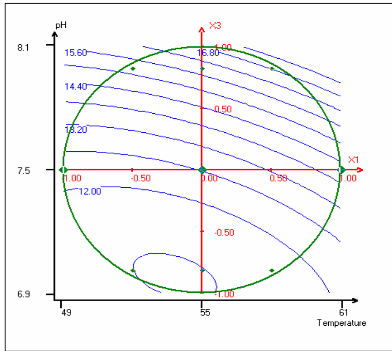
Figure IV.3. Courbes d'isoréponses du degré d'hydrolyse (DH). Tracé du pH en fonction de la température. La valeur du rapport enzyme / substrat (E / S) est maintenue au niveau 0 (centre du domaine expérimental).
