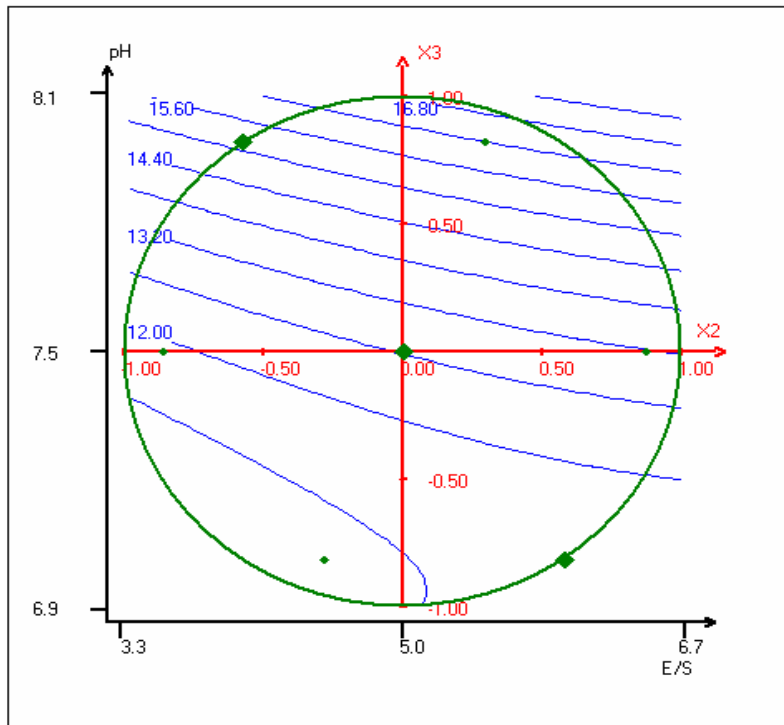
Figure IV.5. Courbes d'isoresponses du degré d'hydrolyse (DH). Tracé du pH en fonction de E / S. La valeur de la température est maintenue au niveau 0 (centre du domaine expérimental).
