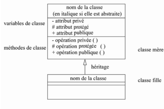
Figure 44– Schéma principal d’une classe en langage UML
