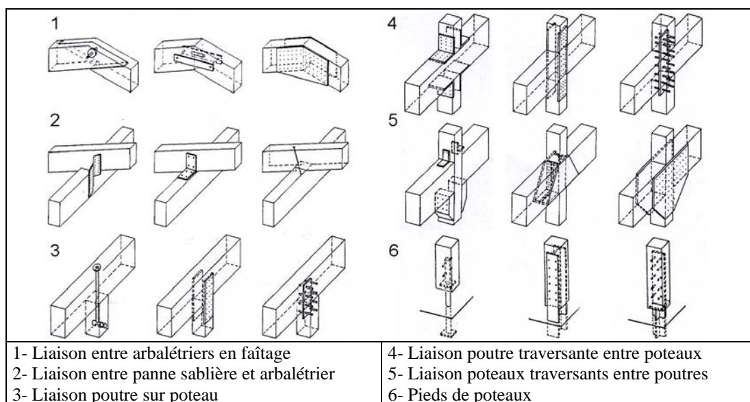
Figure 6– Quelques techniques d’assemblages utilisés dans la construction en bois
