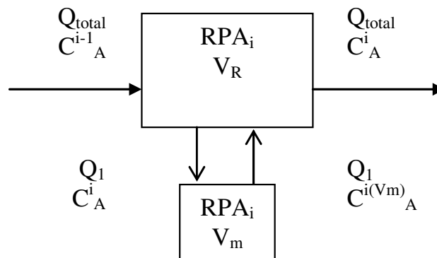
Figure 8 : Représentation d'un RPA i dans la cascade de RPA avec volume stagnant
