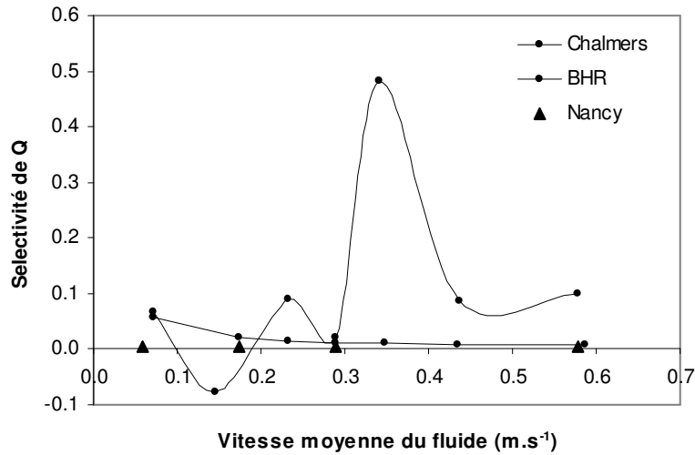
Figure 18 : Validation du modèle de micro-mélange (Évolution de X_Q en fonction de la vitesse moyenne du fluide)
