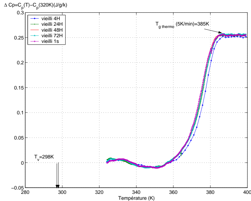
FIG. II.6: Variation de la chaleur spécifique \Delta C_p en fonction de la température ( q=5K/min ) d'un PMMA vieilli à la température ambiante (293K) pour un temps de vieillissement égal à 4H, 24H, 48H, 72H et une semaine
