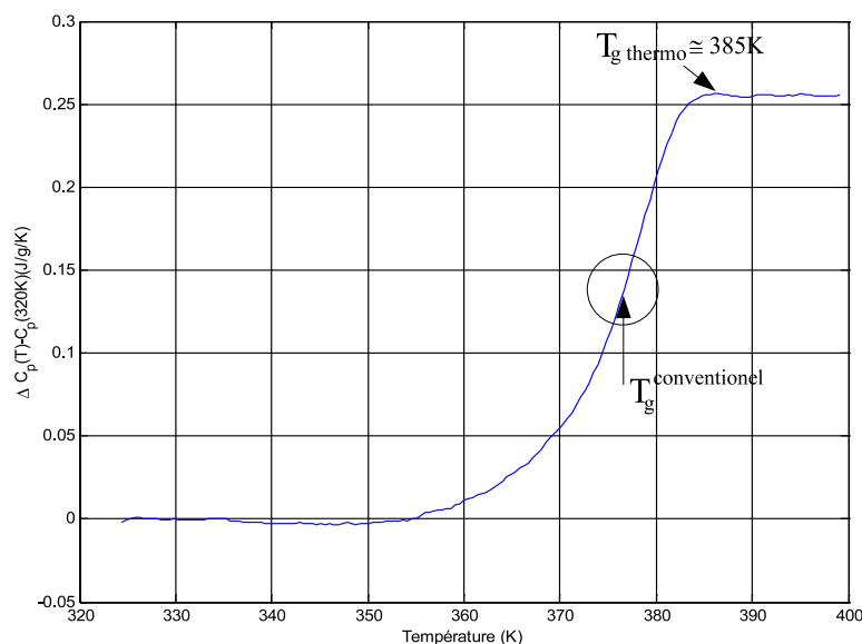
FIG. II.5: Variation de la chaleur spécifique \Delta C_p en fonction de la température ( q=5\text{K/min} ) d'un PMMA dans un état trempé (corrigée)
