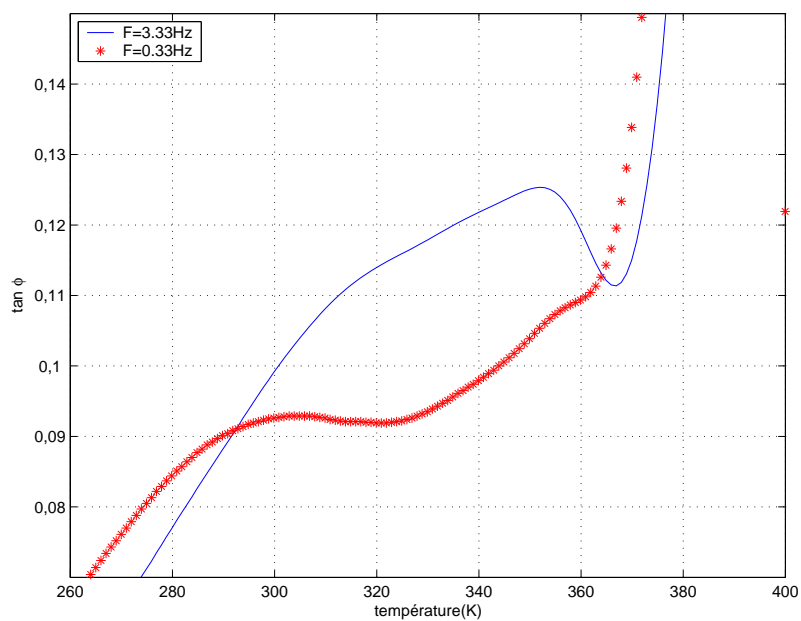
FIG. IV.29: Mesures isochrones à 0,33 (*) et 3,33 (-) Hz de \tan \phi d'un PMMA vieilli 1 semaine à 333 K
