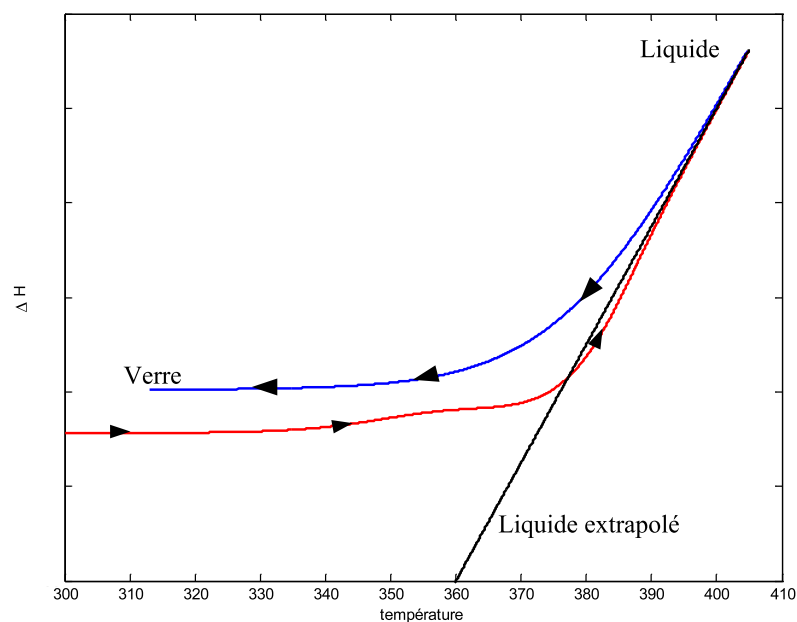
FIG. III.16: Diagramme enthalpique d'un PMMA vieilli 1 semaine à T=313K
