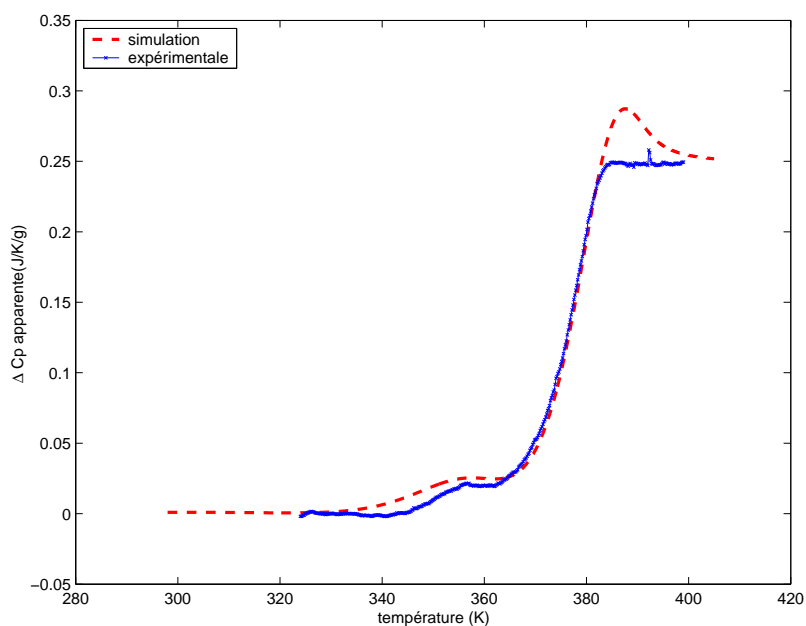
FIG. III.17: \Delta C_p d'un PMMA vieilli 4 heures à 333K : comparaison entre courbe théorique et expérimentale, vitesse de chauffage = 5K/min
