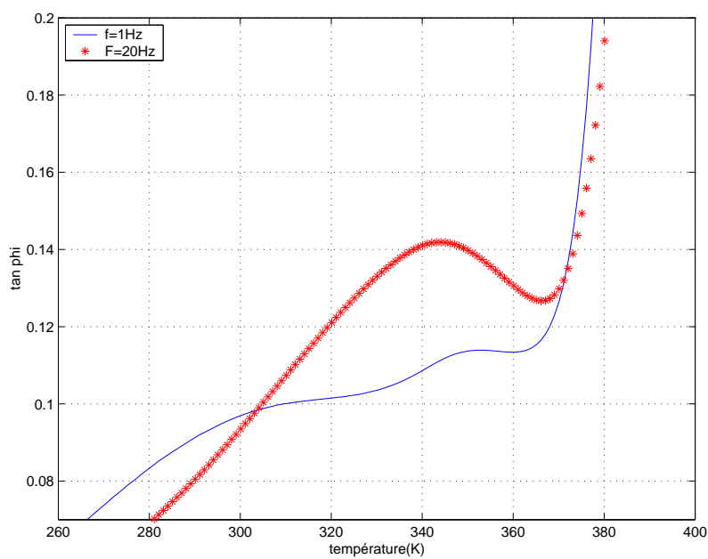
FIG. IV.40: Mesures isochrones à 20 (*) et 1 (-) Hz de \tan \phi d'un PMMA vieilli 1 semaine à 363 K
