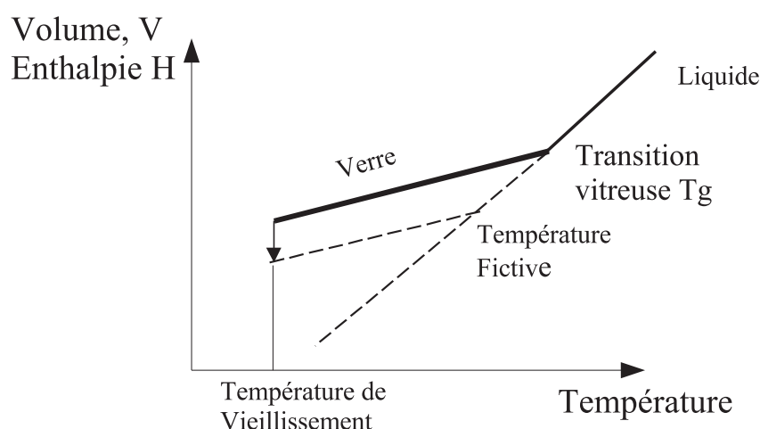
FIG. I.9: Schéma de la dépendance du volume V , et de l'enthalpie H en fonction de la température
