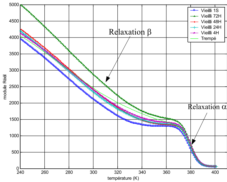
FIG. II.12: Variation du module réel en fonction de la température d'un PMMA vieilli à la température ambiante sollicité à une fréquence F=0,33\text{Hz}
