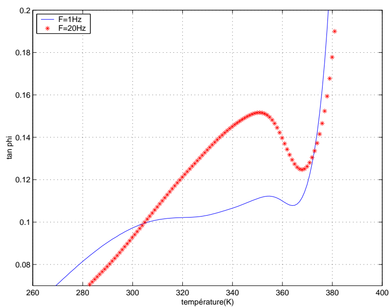
FIG. IV.30: Mesures isochrones à 20 (*) et 1 (-) Hz de \tan \phi d'un PMMA vieilli 1 semaine à 333 K
