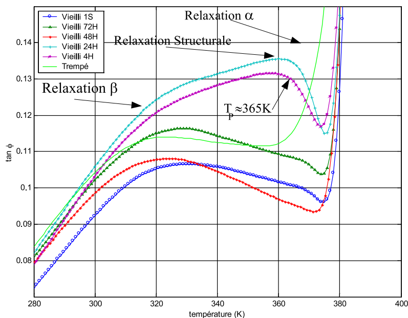
FIG. II.25: Mesure isochrone à 3,33Hz de \tan \phi d'un PMMA vieilli à la température T=363K
