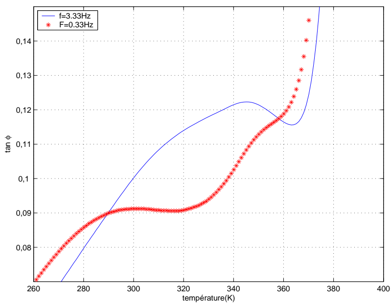
FIG. IV.39: Mesures isochrones à 0,33 (*) et 3,33 (-) Hz de \tan \phi d'un PMMA vieilli 1 semaine à 363 K
