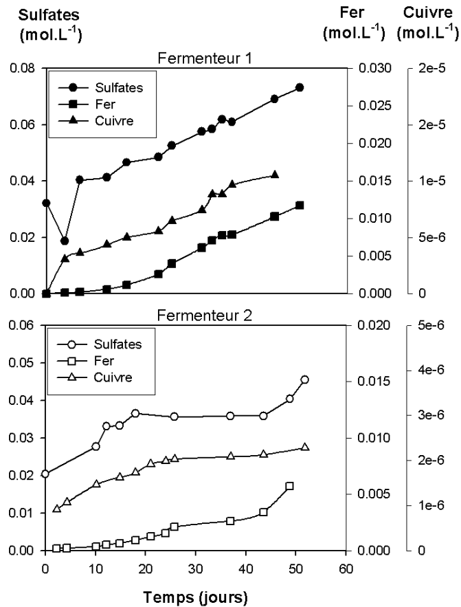
Figure C5. 4 : Suivi des éléments solubilés lors de l'oxydation de la pyrite K par Acidithiobacillus ferrooxidans pour les expériences Ferm1 et Ferm2.
