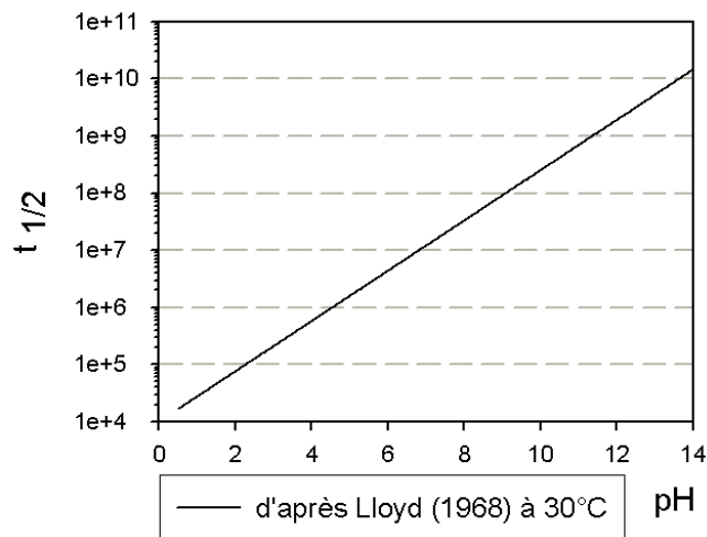
Figure C5. 8 : Evolution du t_{1/2} d'échange (en heures) d'un atome d'oxygène entre un sulfate dissous et une molécule d'eau en fonction du pH, pour une température de 30°C, d'après les données de Lloyd (1968).
