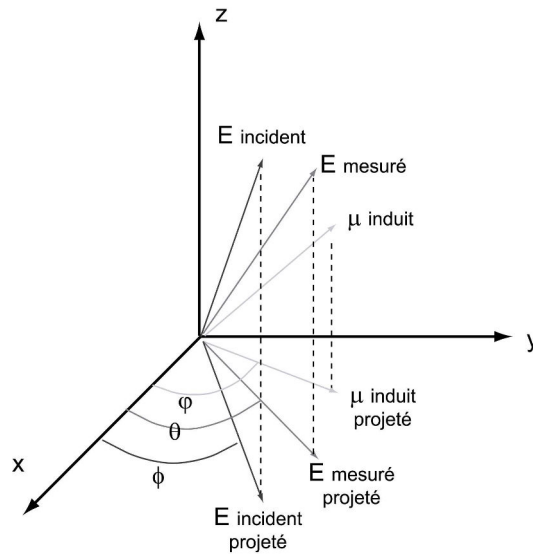
Figure C3. 13 : Grandeurs et orientations du système analysé : x,y,z les orientations cristallines de la pyrite et φ,θ,φ les angles définis par les projections en (x,y) des champs électriques et dipôle induit avec l'axe x.
