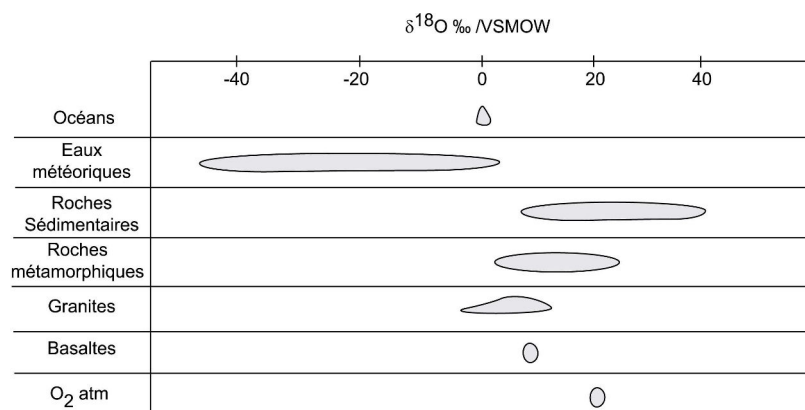
Figure C1. 17 : Composition isotopique en oxygène \delta^{18}\text{O} de différents compartiments terrestres et marins (modified from Clark and Fritz, 1997).
