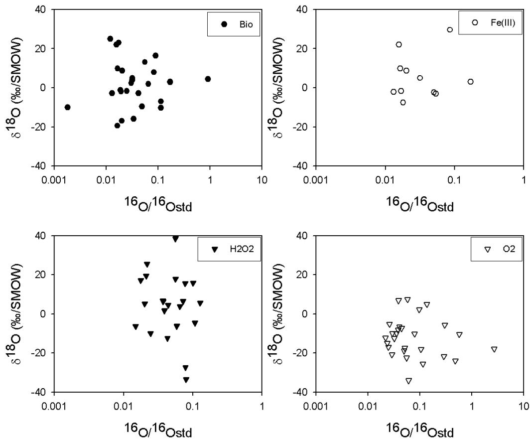
Figure C5. 16 : Répartition des compositions isotopiques en oxygène des produits d'altération en surface de grains de pyrite en fonction de l'agent oxydant : biologique, ions ferriques, peroxyde d'hydrogène, témoins d'oxydation à l'air libre.
