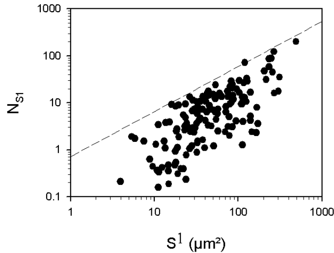
Figure C4.19 : Corrélation entre le nombre de bactéries adhérentes dans les figures de corrosion et la taille de ces figures de corrosion ( \mu\text{m}^2 ) pour toutes les points d'observation.
