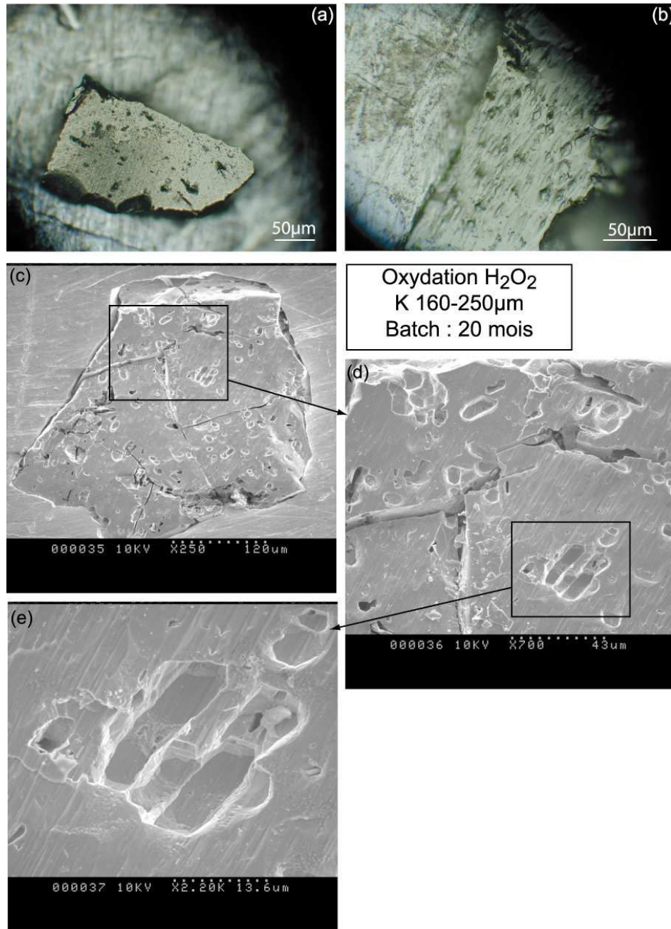
Figure C4. 2 : Images d'une surface de pyrite oxydée par traitement abiotique H_2O_2 pendant 20 mois. (a) et (b) : photographie en microscopie optique (x200) ; (c), (d) et (e) : images MEB.
