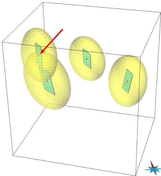
(b) SSZ à \beta = 0.5 : non-respect des contraintes de SSZ
