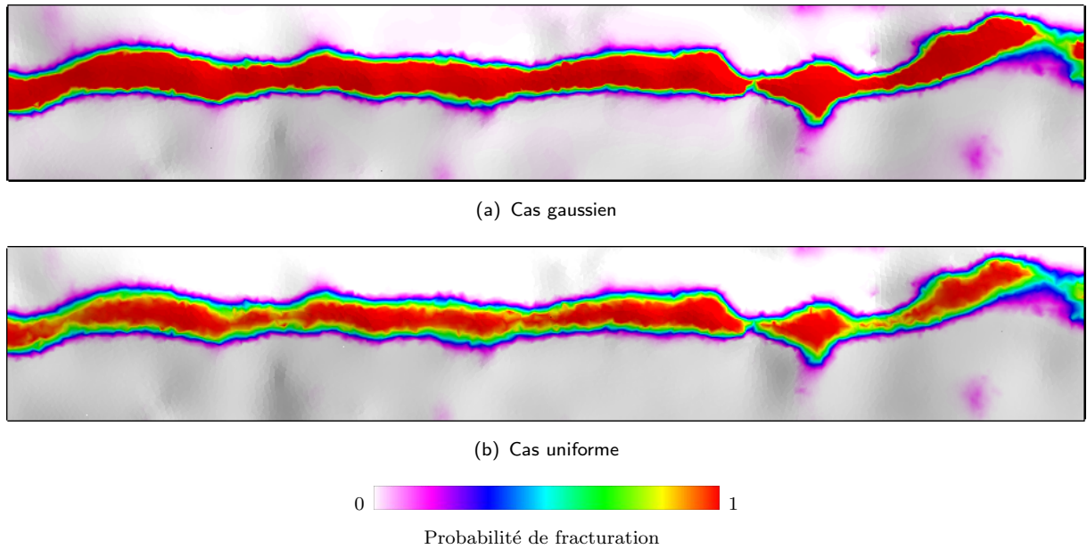
Fig. II.16: Comparaison des probabilités de fracturation pour les cas gaussien et uniforme. Vue de dessus.
