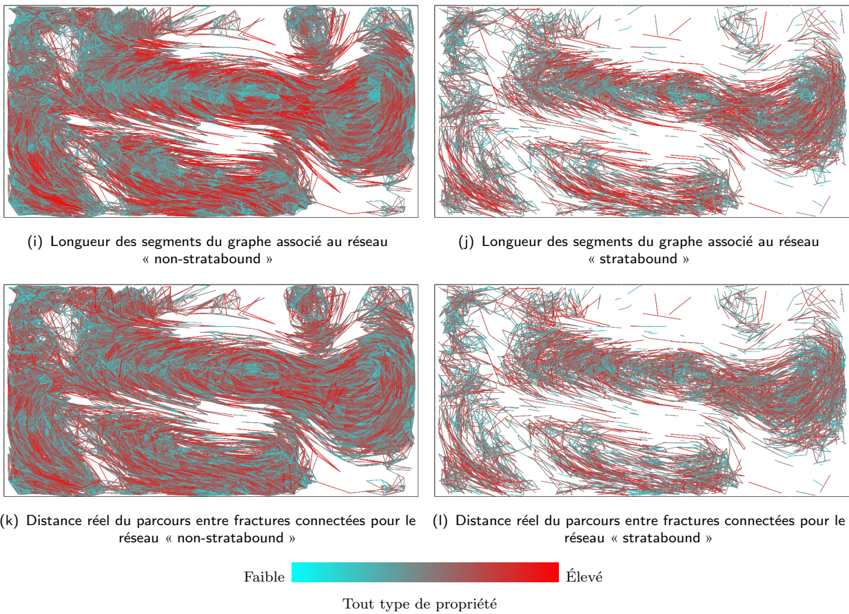
Fig. IV.11: Impact des contraintes géologiques sur la connectivité d'un réseau de fractures discrètes. Des propriétés sont calculées sur deux réseaux, l'un « non-stratabound » et l'autre « stratabound ».
