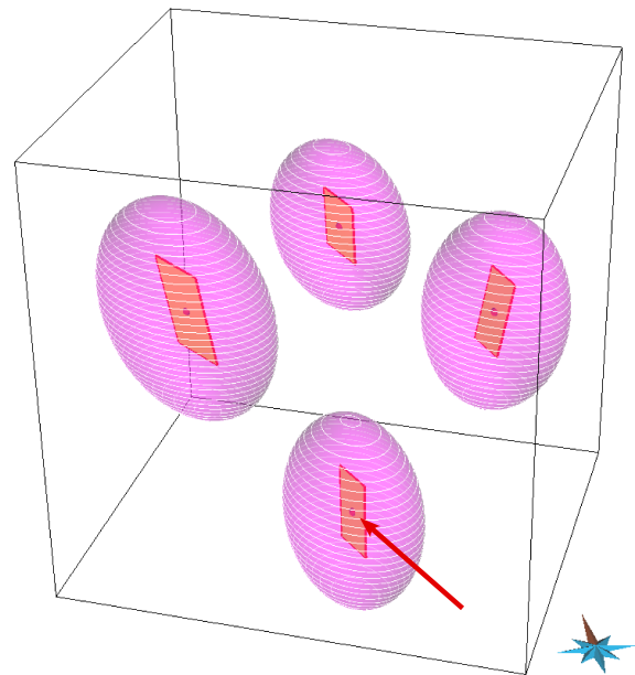
(c) SSZ à \beta = 0.5 : respect des contraintes de SSZ
