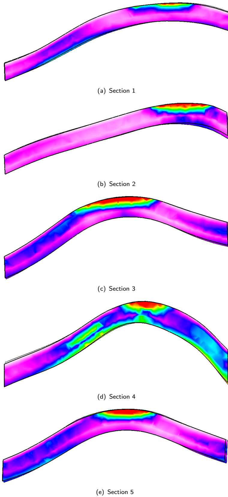
Fig. II.18: Probabilité de fracturation représentée sur un ensemble de sections bidimensionnelles effectuées du Sud (Section 1) vers le Nord (Section 5). Le Nord est représenté par la flèche bleue de la rosace située en bas et à droite sur la figure II.17.
