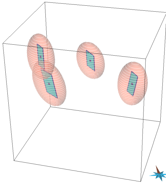
(a) SSZ à \beta = 0.1 : respect des contraintes de SSZ
