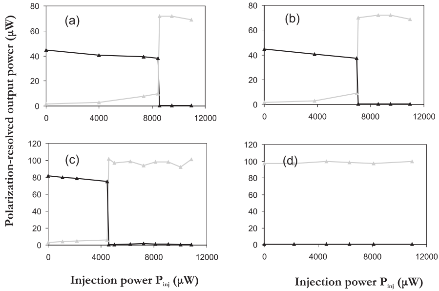
Figure B.3.2: Evolution de la puissance de sortie des modes basse fréquence BF ( x -polarisation horizontale en noir) et haute fréquence HF ( y -polarisation verticale en gris) du VCSEL 2 lorsqu'on varie la puissance injectée P_{inj} pour deux valeurs distinctes de courant d'injection I_{SL} : I_{SL} = 1.9 \text{ mA} et detuning \Delta\nu = -36 \text{ GHz} : (a) P_{inj} croissant, (b) P_{inj} décroissant ; I_{SL} = 2.603 \text{ mA} et detuning \Delta\nu = -20 \text{ GHz} : (c) P_{inj} croissant, (d) P_{inj} décroissant.
