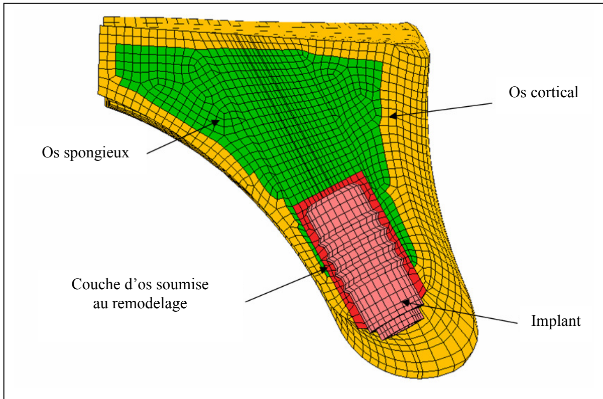
FIG.4.11 : Coupe du modèle II avec les matériaux constituants.
