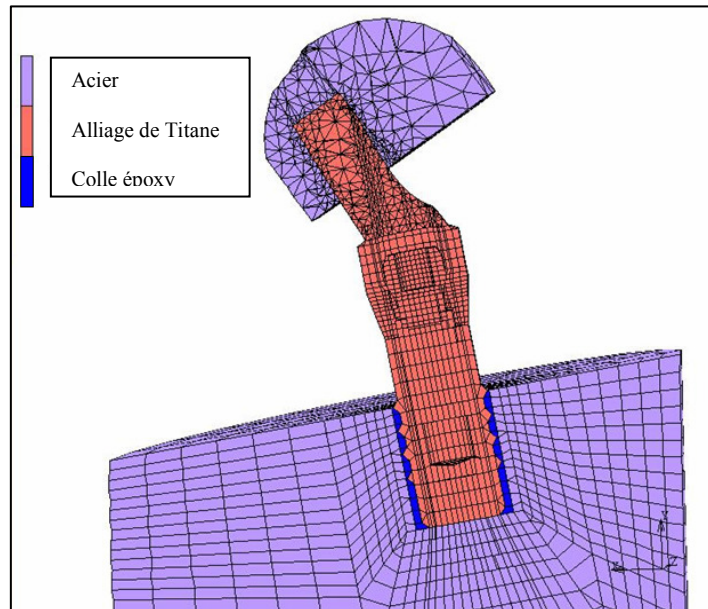
FIG 4.6 : Coupe du modèle complet avec les matériaux constituants
