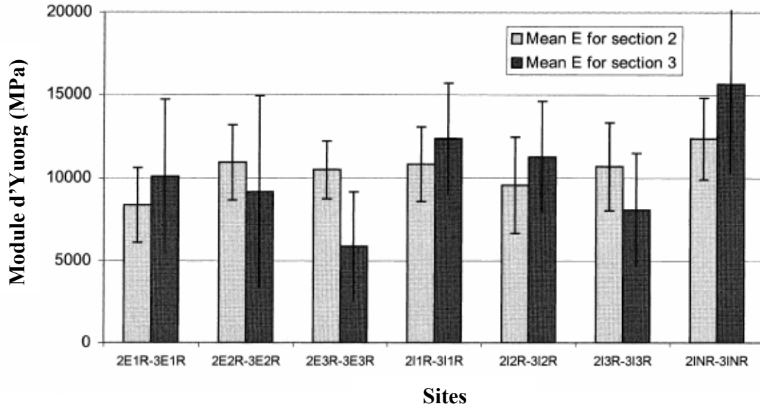
FIG.3.4 : Module d'Young en fonction des sites (section 2 : molaire, section 3 : prémolaire, E : externe, I : interne, L : gauche, R : droite) (d'après Lettry et al.2003 [3.23]).
