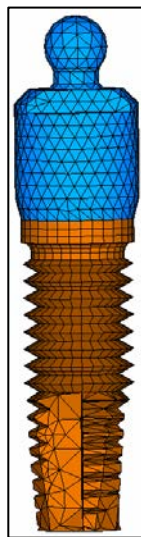
FIG.5.14 : Maillage : implant et partie mâle de l'attache.
