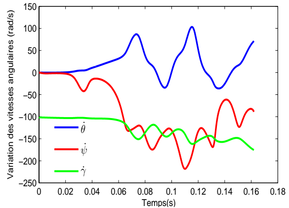
FIGURE 5.2: Convergence des vitesses longitudinales, de roulis et de rotation du rotor principal
