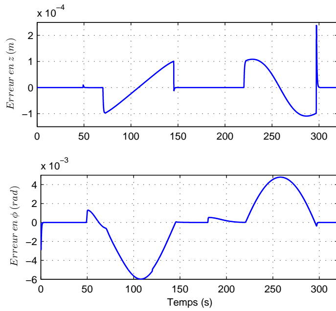
FIGURE 4.21: Erreur de suivi en z et en \phi
