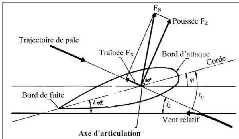
FIGURE 2.14: Profil d'une pale d'hélicoptère [6]
