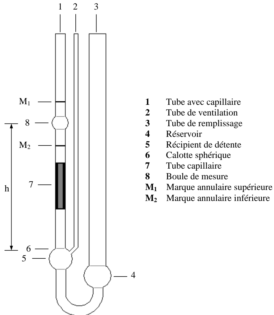
Schéma A-4 : Représentation d'un microviscosimètre de Ubbelohde
