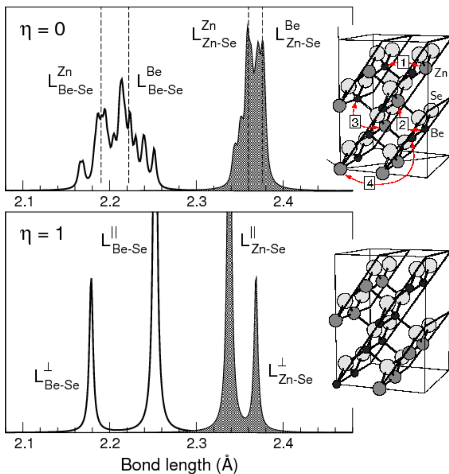
FIG. A-3 – Distributions des longueurs de liaison Zn-Se et Be-Se, élargies à mi-hauteur de 0.0025 \text{ \AA} , de l'alliage aléatoire ZnBeSe 2 ( \eta = 0 , panneau supérieur) et totalement ordonné de type CuPt ( \eta = 1 , panneau inférieur), calculées à partir des supercellules montrées sur la droite. La dénomination des différentes structures est tirée du modèle de percolation à \eta = 0 et de la terminologie usuelle dans le cas d'un super-réseau ( \eta = 1 ). Les valeurs finies de \eta de 0.25, 0.50 et 0.75 sont obtenues en cumulant les échanges de paires Zn \leftrightarrow Be numérotés de 1 à 4 comme il est indiqué dans la supercellule supérieure.
