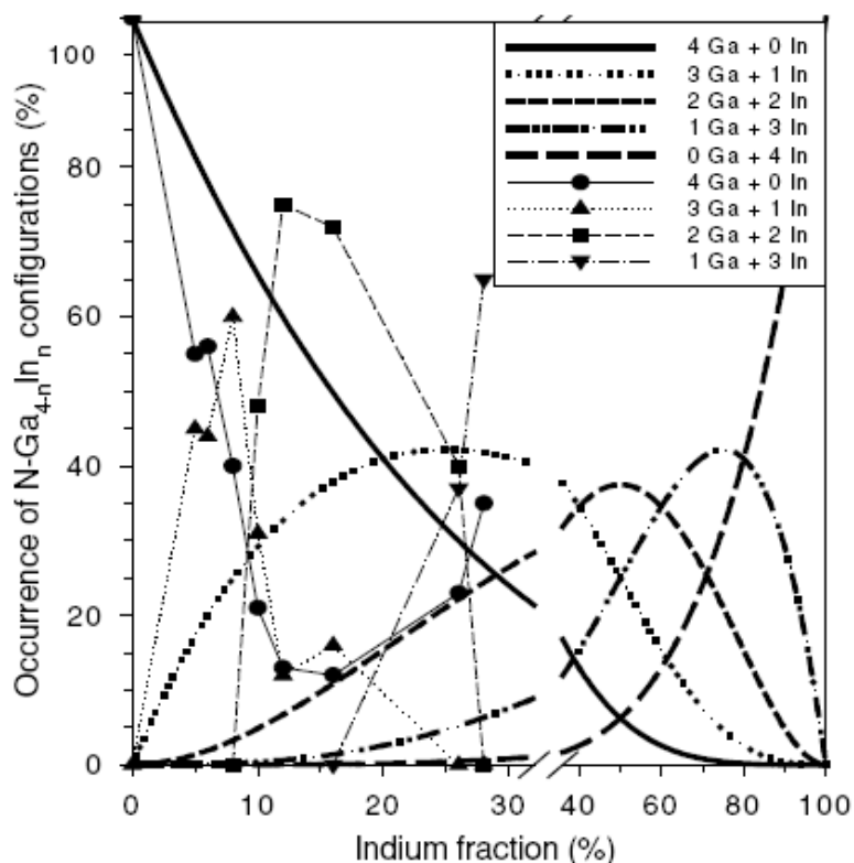
FIG. III-14 – Population des différents clusters de type N-Ga 4-n In n en fonction de la fraction d’In dans les couches épitaxiales de In y Ga 1-y As 1-x N x ( x \sim 2\% ). Les symboles connectés par les traits fins correspondent à des estimations expérimentales après recuit des couches à 800 °C pendant 30 sec. (jusqu’à 28%In). Les tracés épais correspondent à des tendances théoriques obtenues sur la base d’une substitution aléatoire de l’azote, du gallium et de l’indium sur les sites du réseau. La figure est extraite de Alt et al. (2006).
