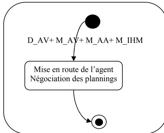
Statechart 4.3 : Activation de l'ANP
