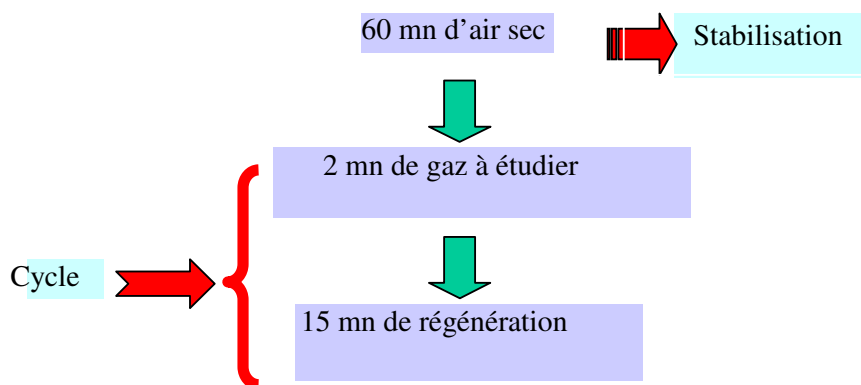
Figure V-4 : Cycle de mesures pour les capteurs polymères
