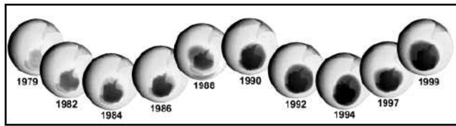
Figure I-5 : Evolution du trou de la couche d'ozone de 1979 à 1999
