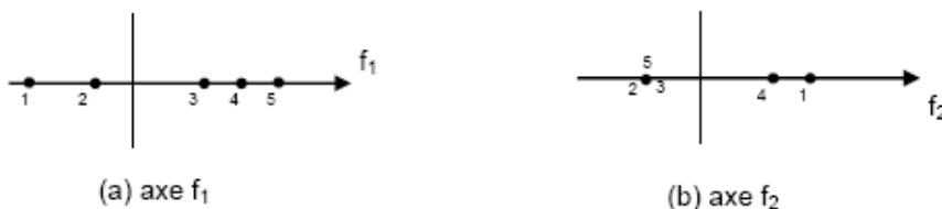
Figure VII-3 : Projections des points sur f_1 et f_2
