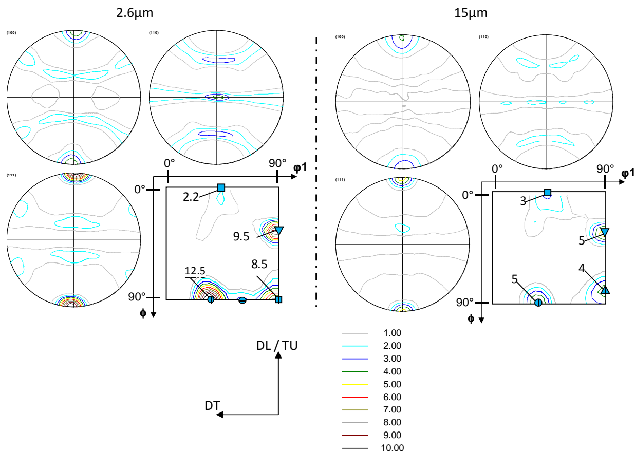
Figure 3.25 Figures de pôles recalculées \{100\}\{110\}\{111\} et sections à \varphi_2=45^\circ de la FDO relatives aux matériaux à petits et gros grains (respectivement 2.6\mu\text{m} et 15\mu\text{m} ), déformés en traction DL à 0.52 de déformation vraie.
