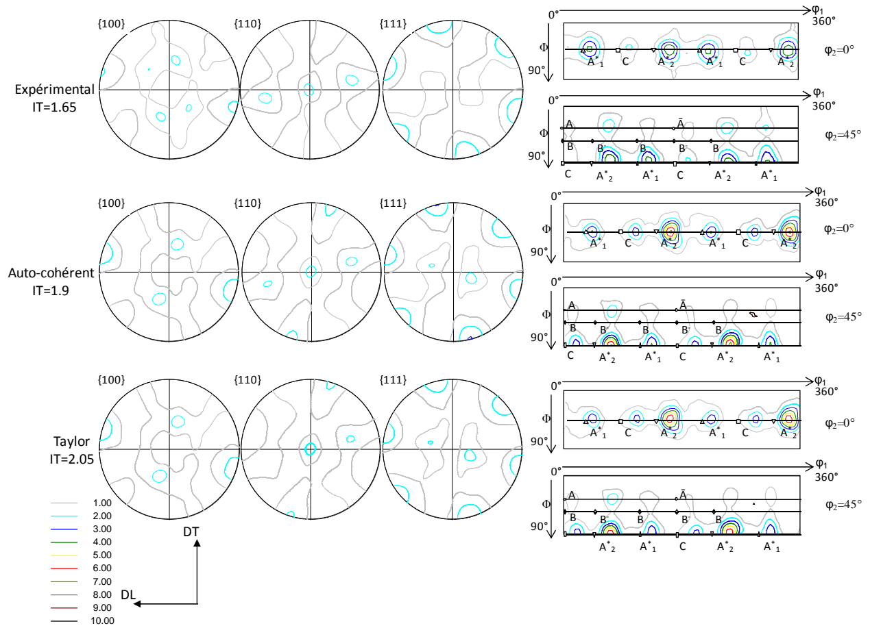
Figure 5.21 Textures expérimentale et simulées lors d'un essai de cisaillement réversible à +0.06 / -0.2 de déformation équivalente.
