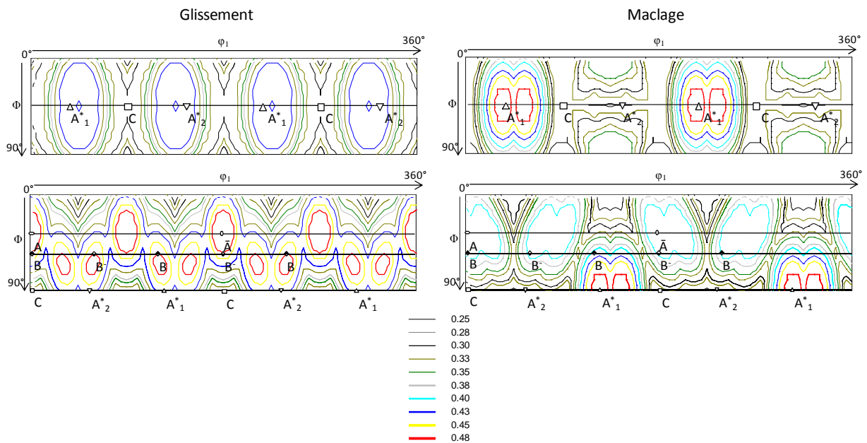
Figure 4.6 : Sections à \phi_2=0^\circ et \phi_2=45^\circ représentant les lignes d'iso-densités des facteurs d'orientation maximum pour le glissement négatif.
