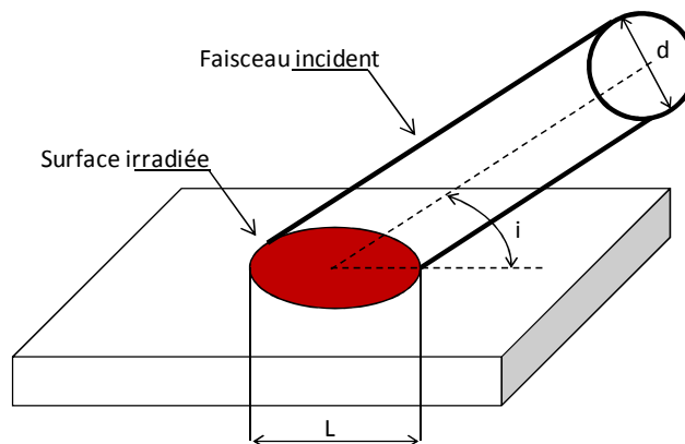
Figure A.2 Géométrie de la surface irradiée pour un collimateur cylindrique ( d : diamètre du collimateur ; longueur du grand axe : L ; angle réel d'incidence : i ).
